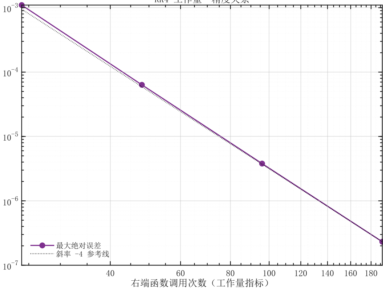
RK4 工作量—精度关系
