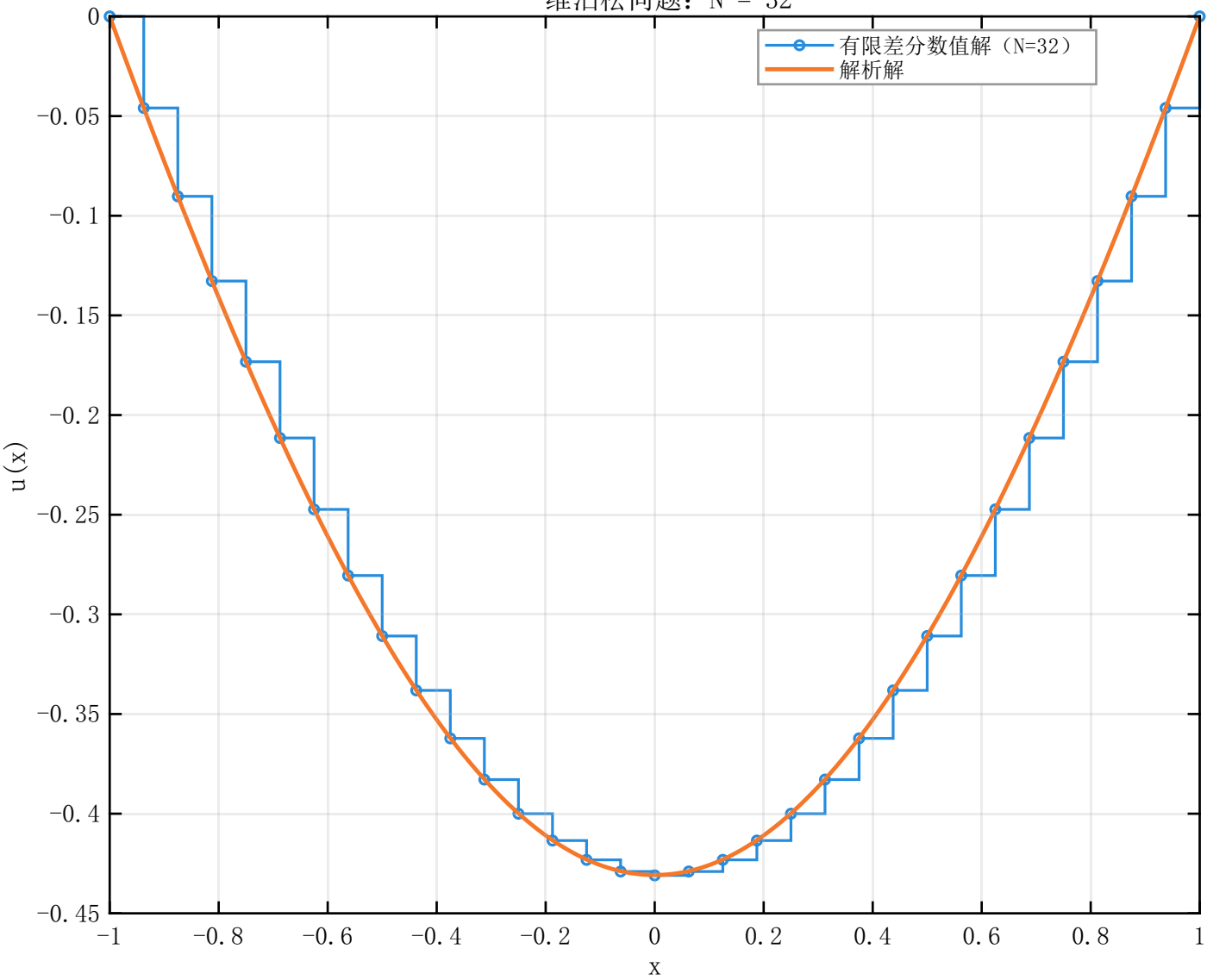
一维泊松问题: N = 32
