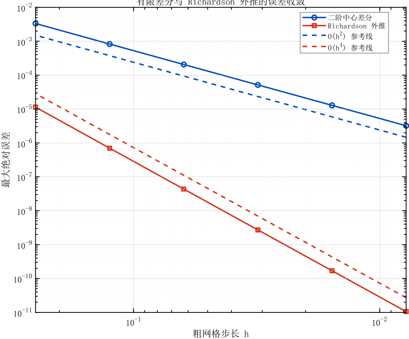
有限差分与 Richardson 外推的误差收敛
