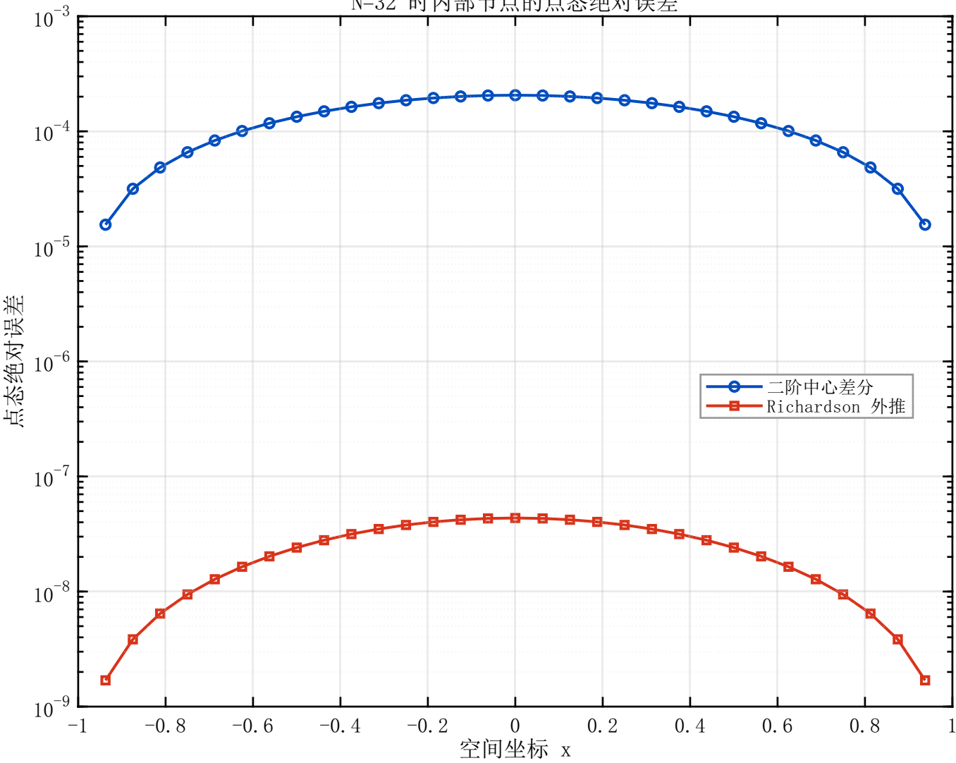
N=32 时内部节点的点态绝对误差
