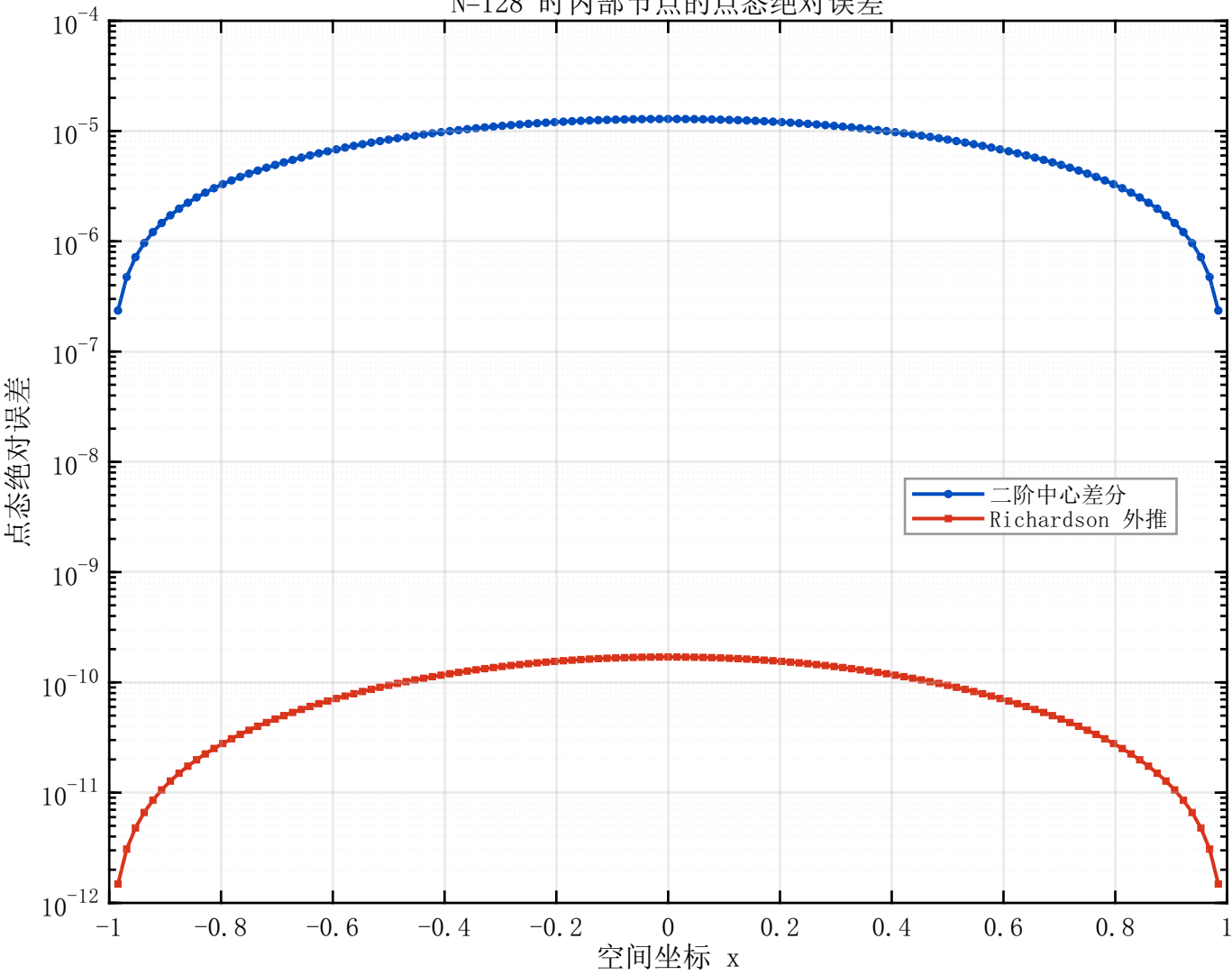
N=128 时内部节点的点态绝对误差
