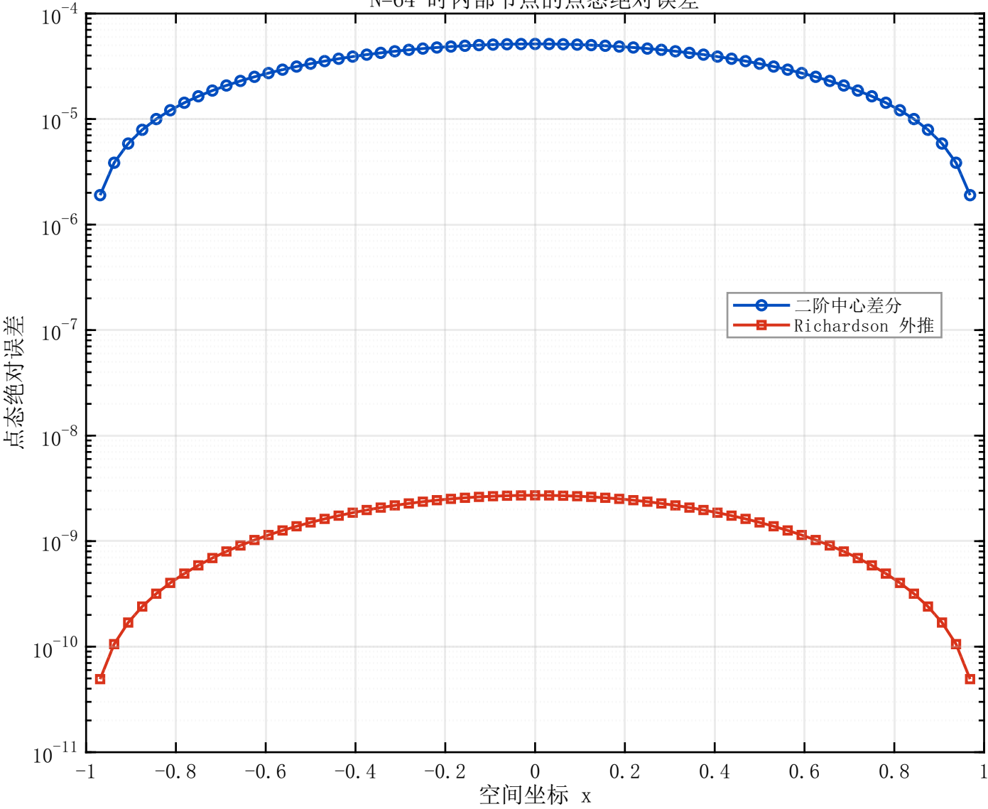
N=64 时内部节点的点态绝对误差
