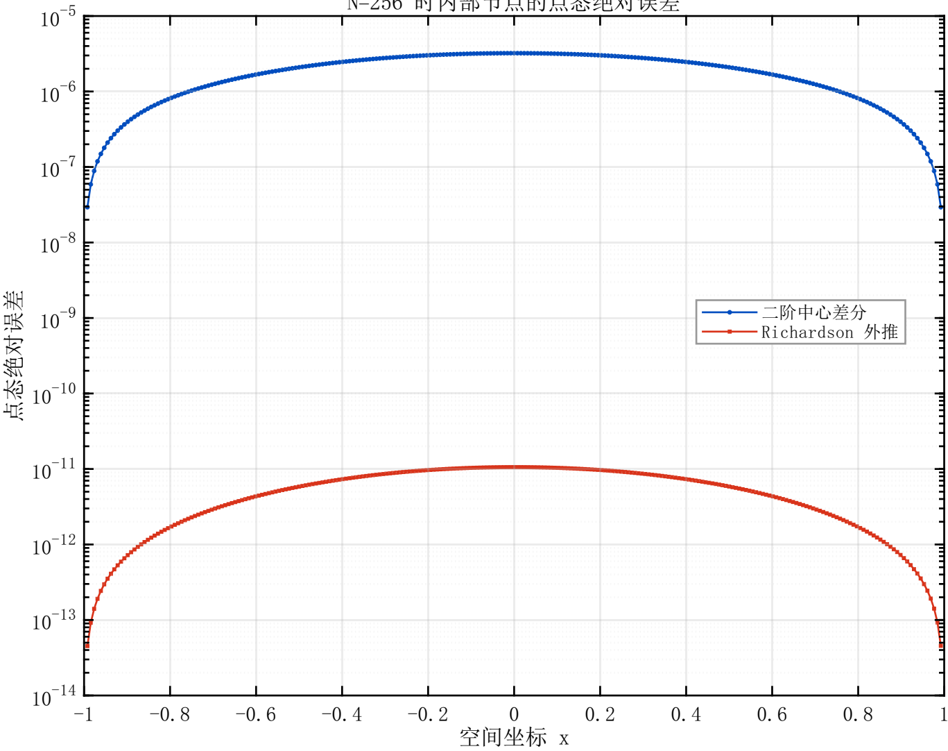
N=256 时内部节点的点态绝对误差
