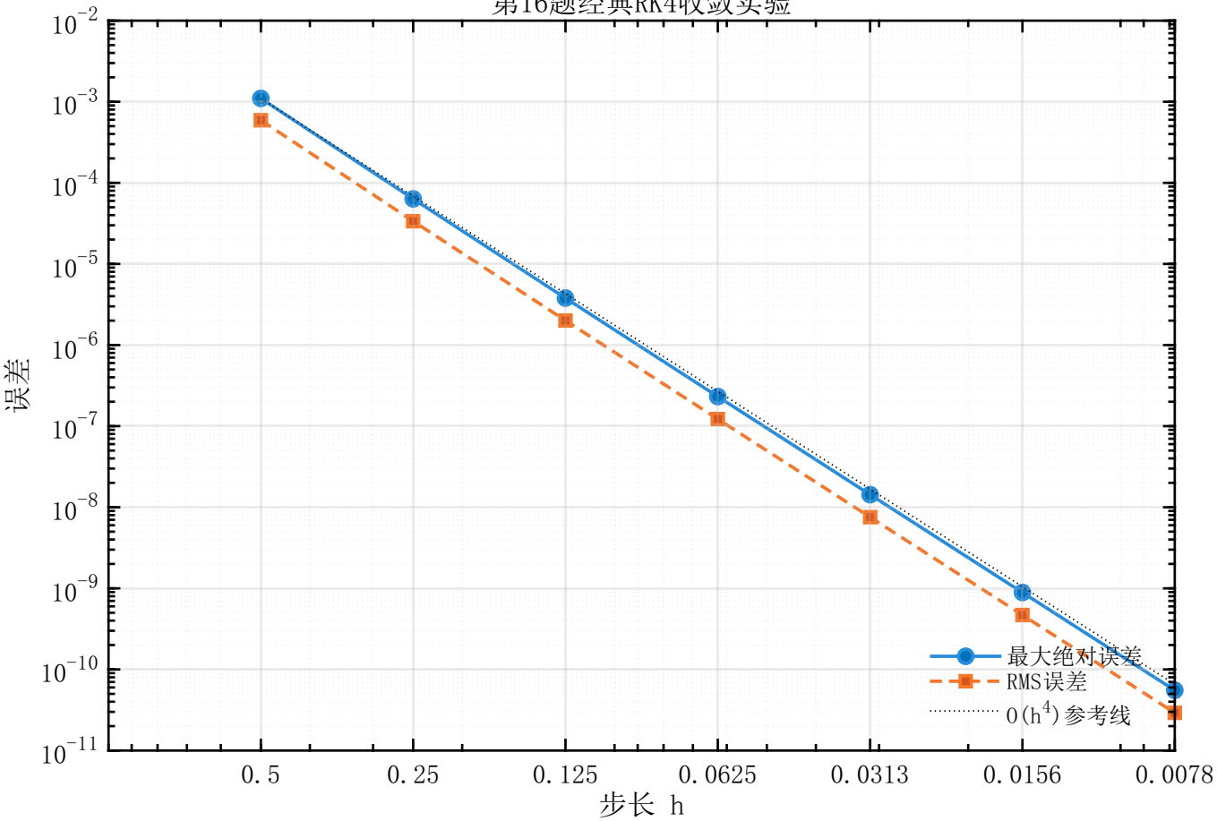
第16题经典RK4收敛实验
