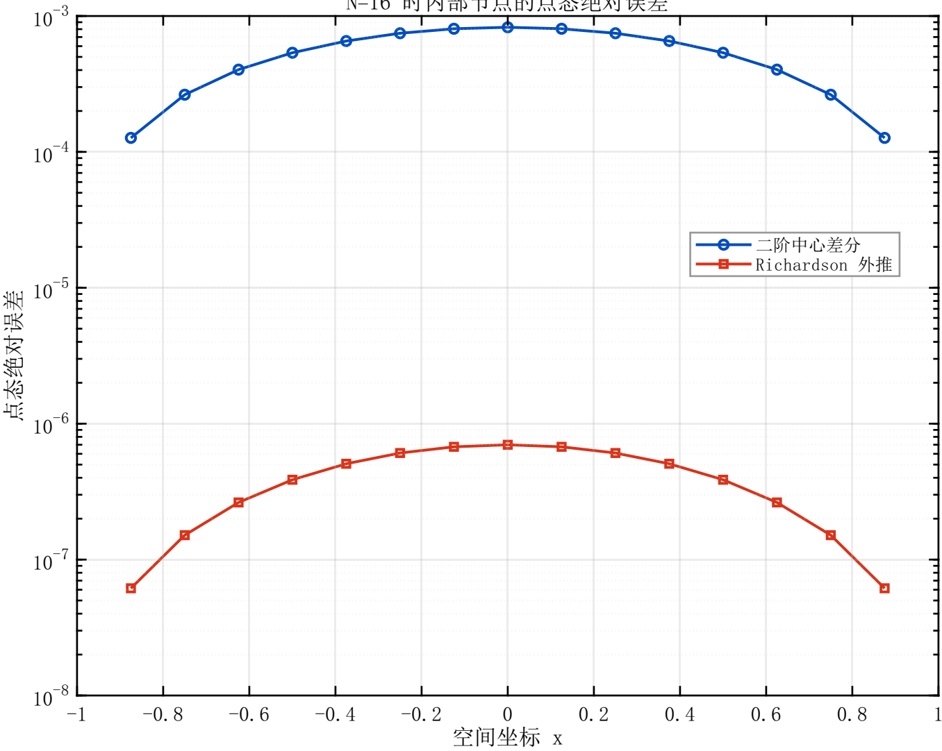
N=16 时内部节点的点态绝对误差
