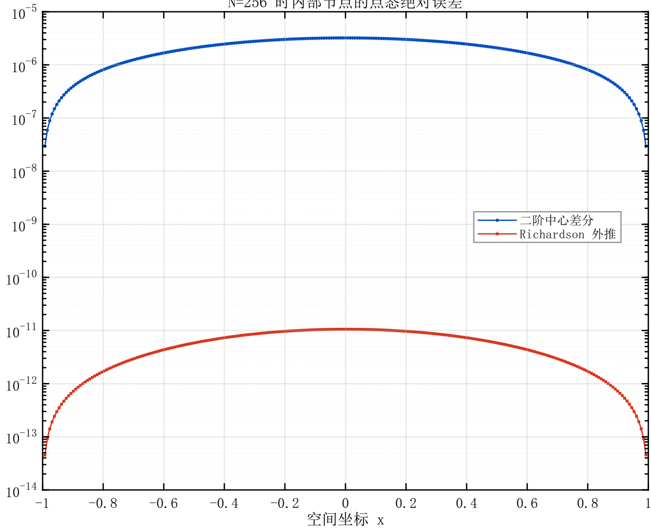
N=256 时内部节点的点态绝对误差
