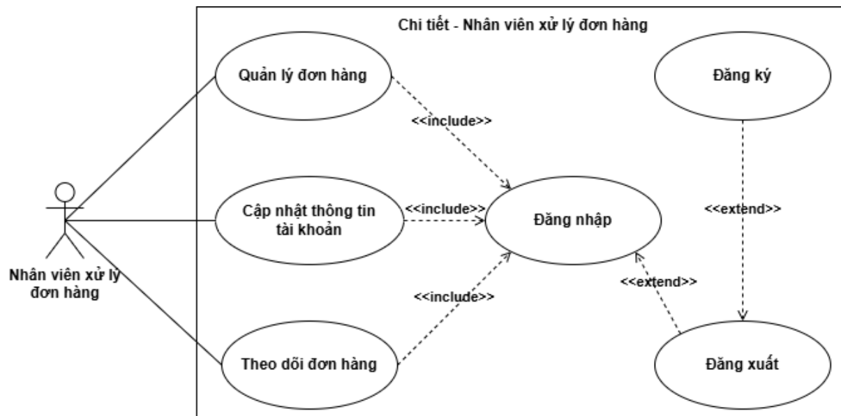
Hình 5: Biểu đồ ca sử dụng Nhân viên xử lý đơn hàng
