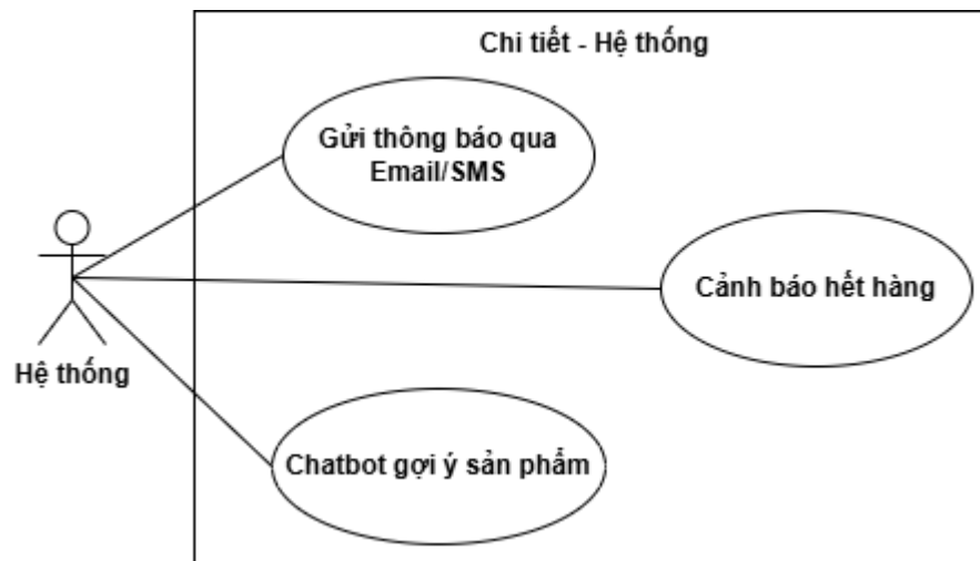
Hình 10: Biểu đồ ca sử dụng Hệ thống
