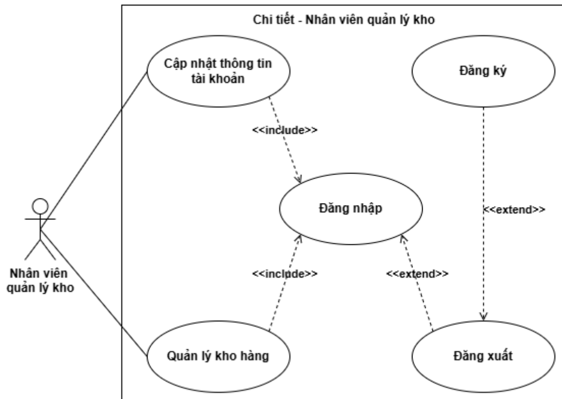
Hình 4: Biểu đồ ca sử dụng Nhân viên quản lý kho
