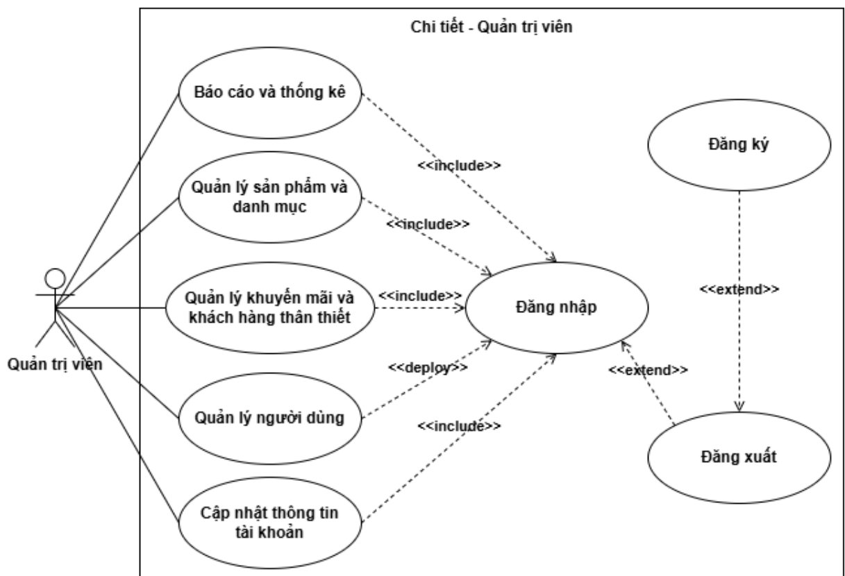
Hình 8: Biểu đồ ca sử dụng Quản trị viên
