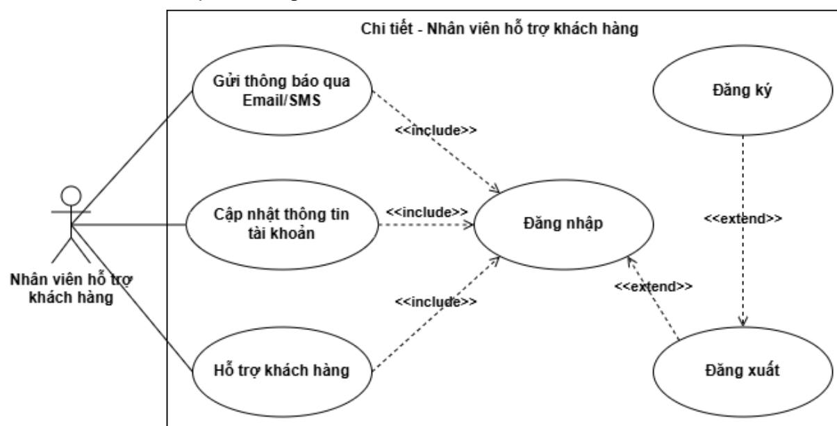
Hình 6: Biểu đồ ca sử dụng Nhân viên hỗ trợ khách hàng
