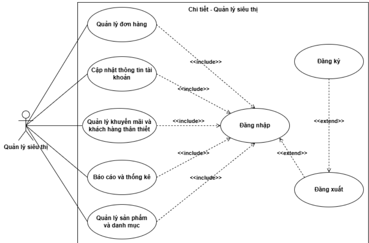
Hình 3: Biểu đồ ca sử dụng Quản lý siêu thị
