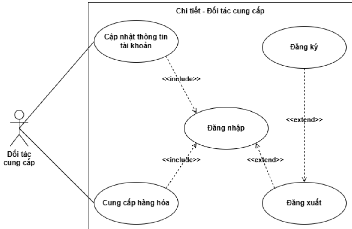
Hình 7: Biểu đồ ca sử dụng Đối tác cung cấp
