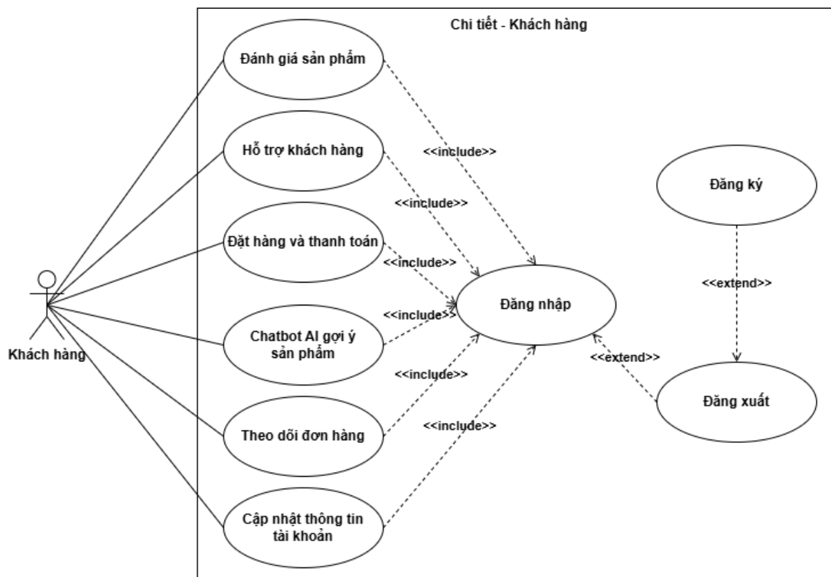
Hình 2: Biểu đồ ca sử dụng Khách hàng
