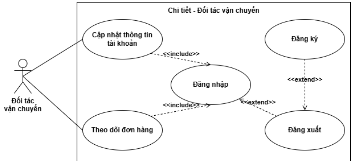
Hình 9: Biểu đồ ca sử dụng Đối tác vận chuyển
