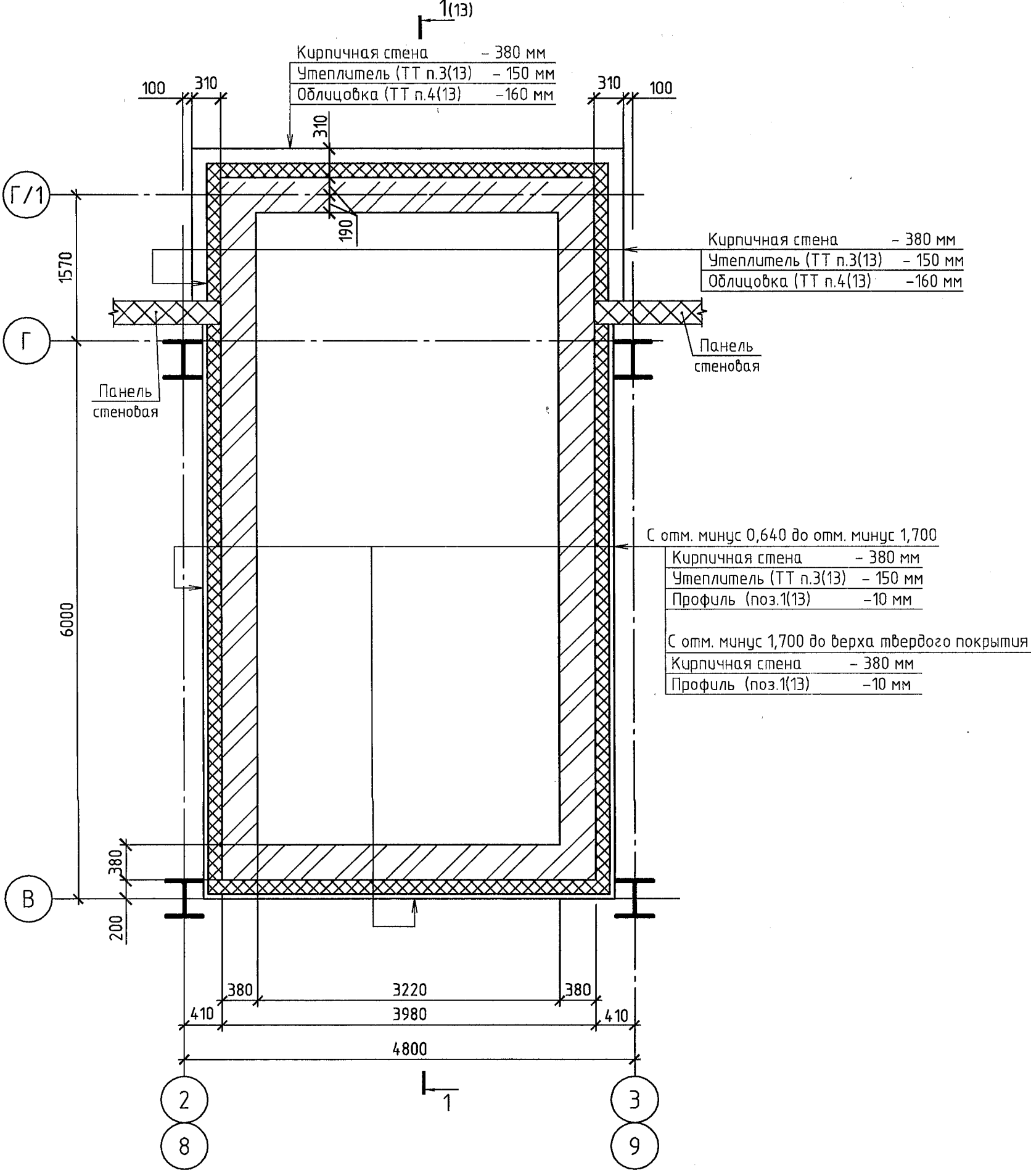
Схема расположения утепления лестниц Л1 ниже отм. 0,000
