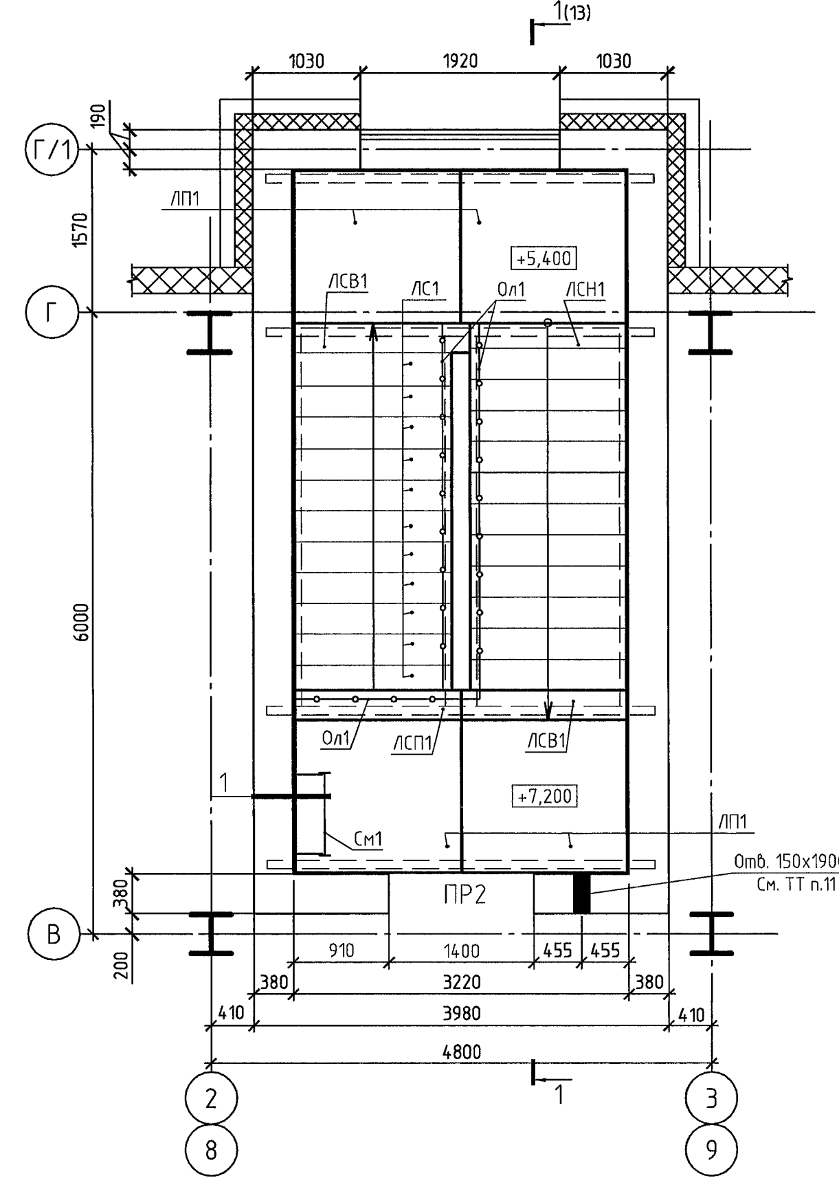
Схема расположения элементов лестниц Л1 на отм. +7,200
