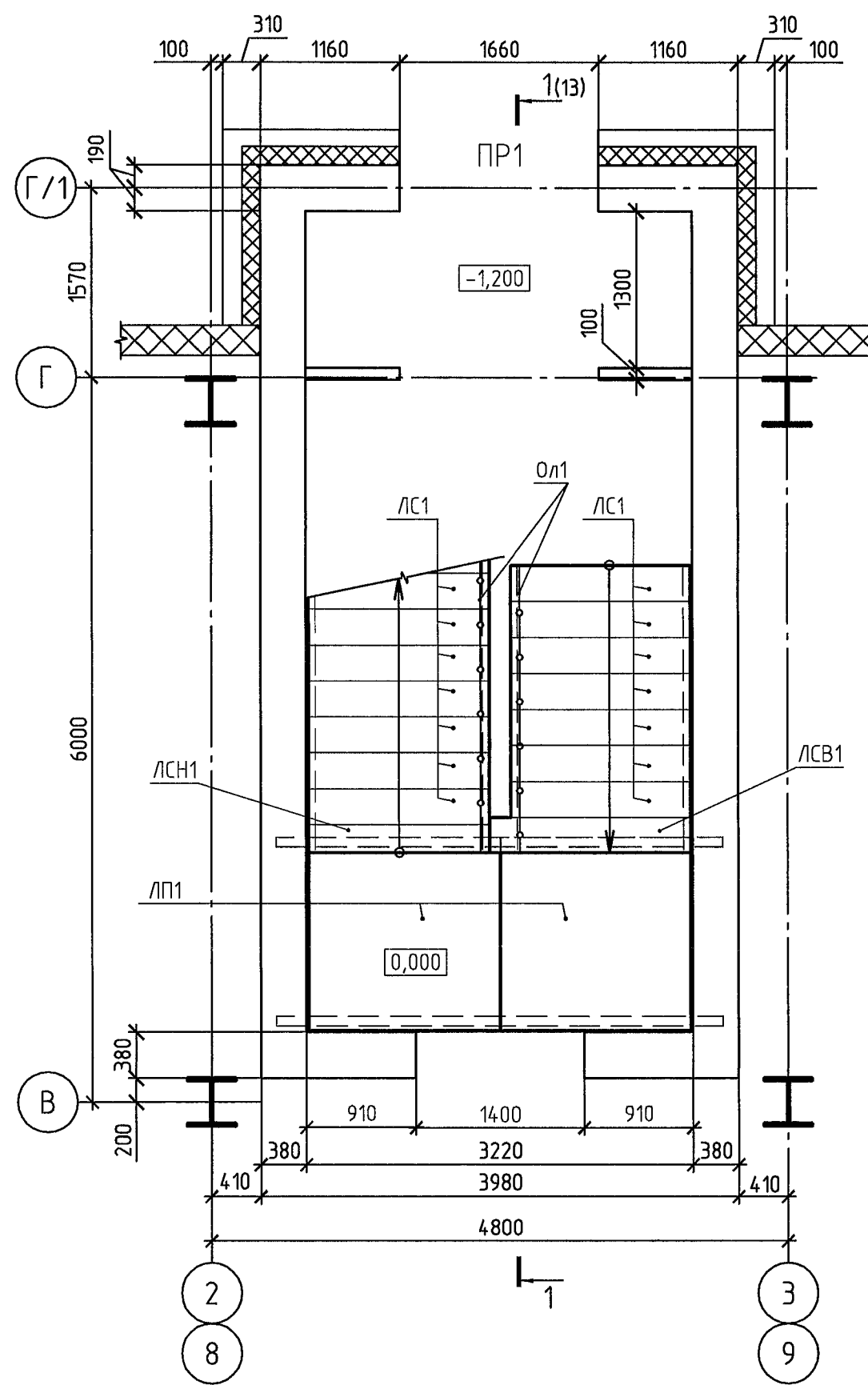
Схема расположения элементов лестниц Л1 на отм. 0,000
