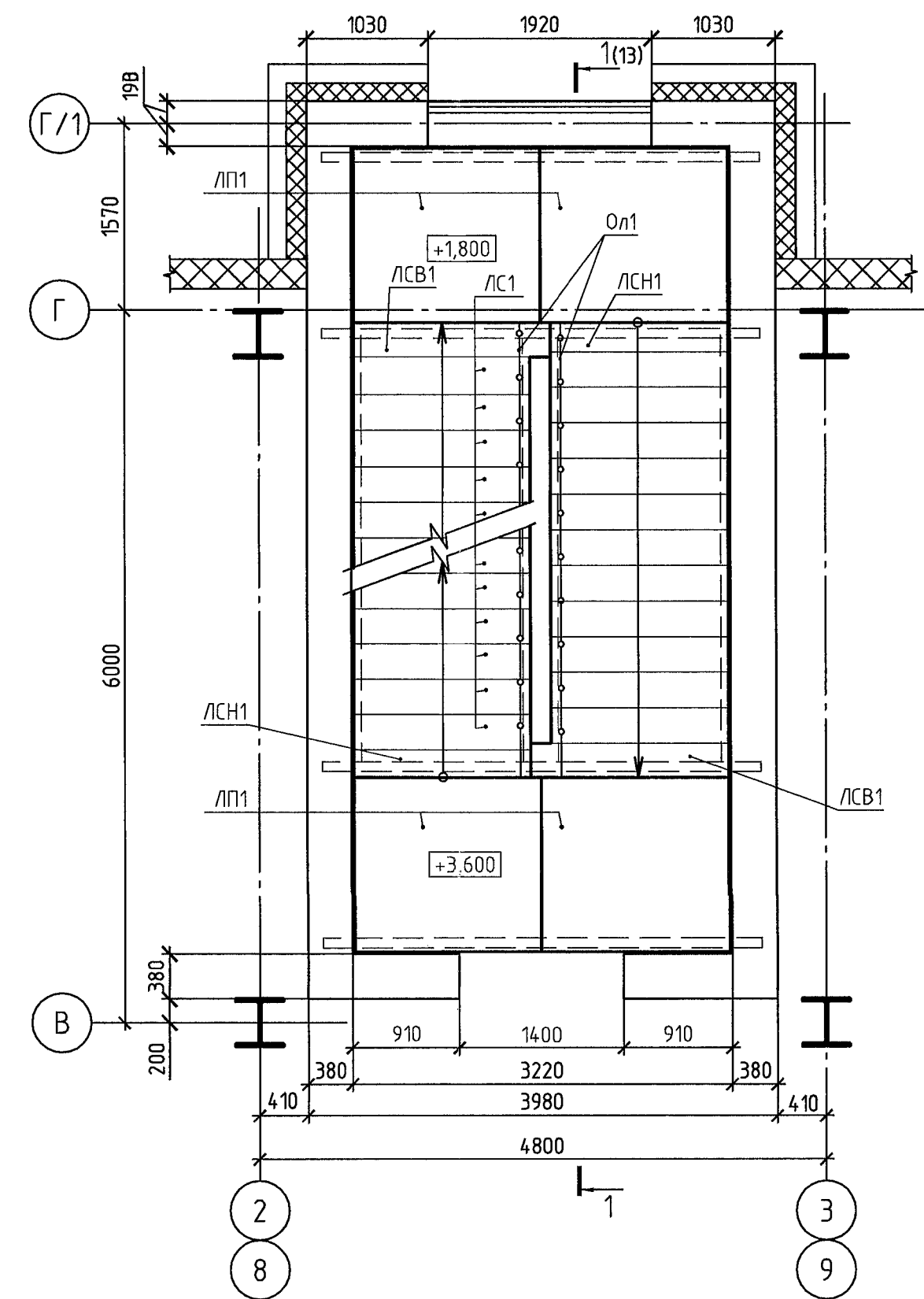
Схема расположения элементов лестниц Л1 на отм. +3,600
