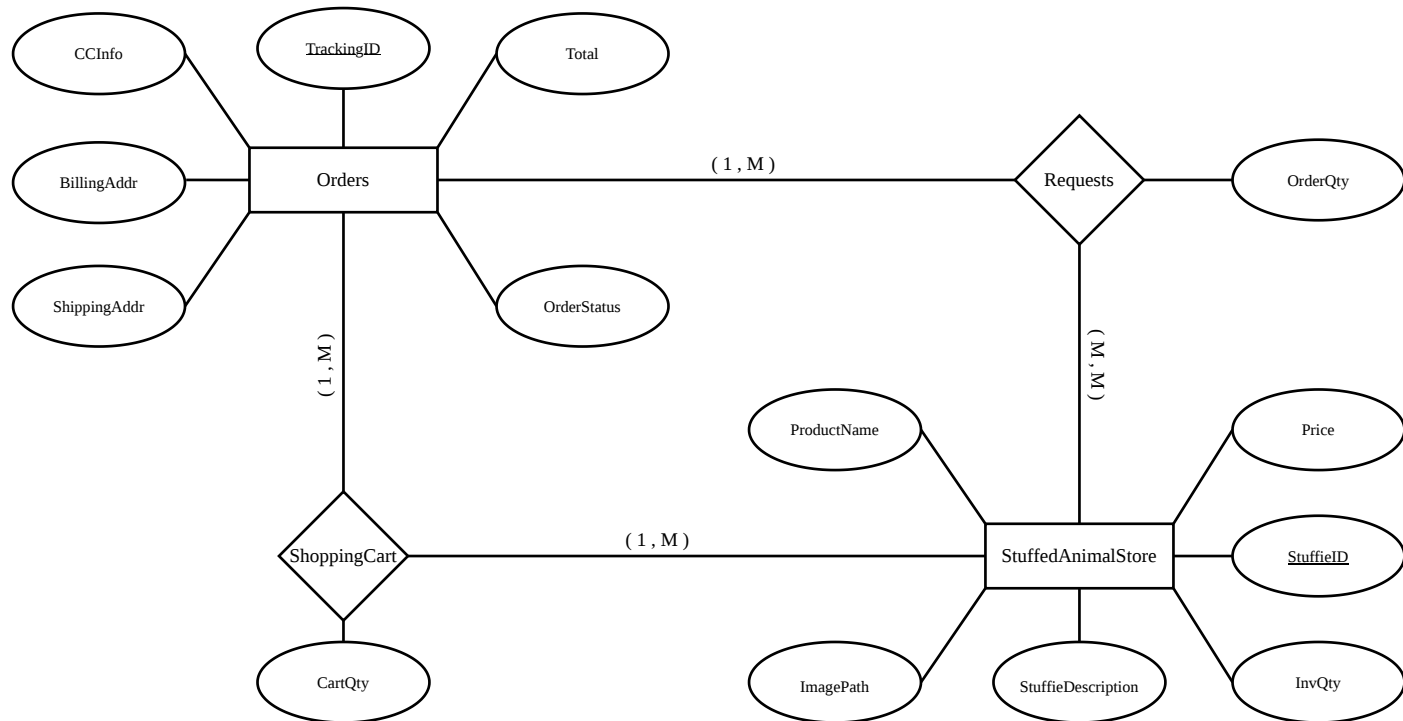
ER Diagram
