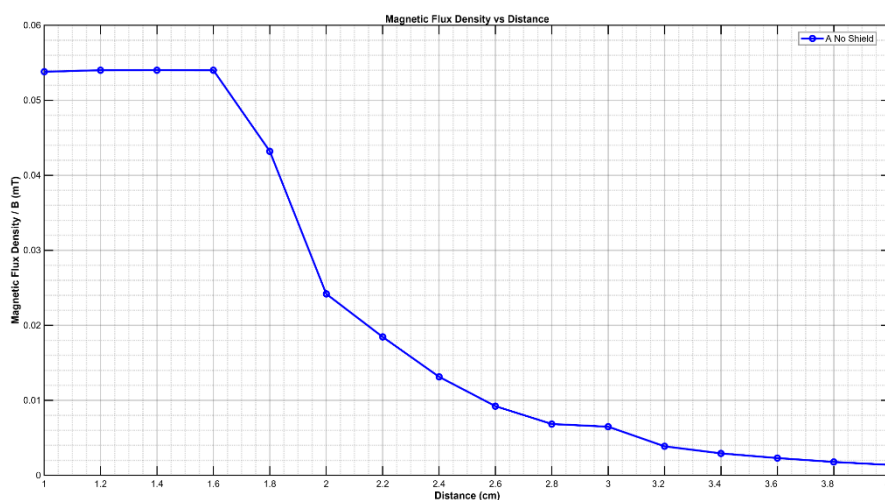
ภาพ 8 กราฟขั้ว A กรณี No Shield
