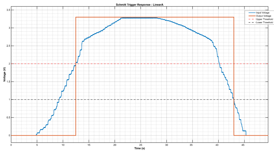
ภาพ 3 Linear potentiometer A
