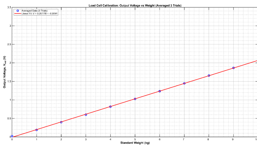
ภาพ 20 กราฟแสดงการ calibration
