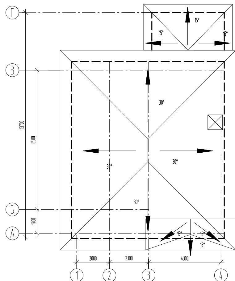
ПЛАН КРОВЛИ
