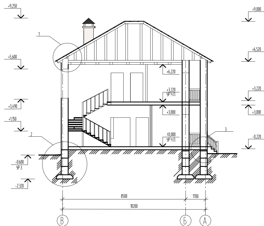
РАЗРЕЗ 1-1
