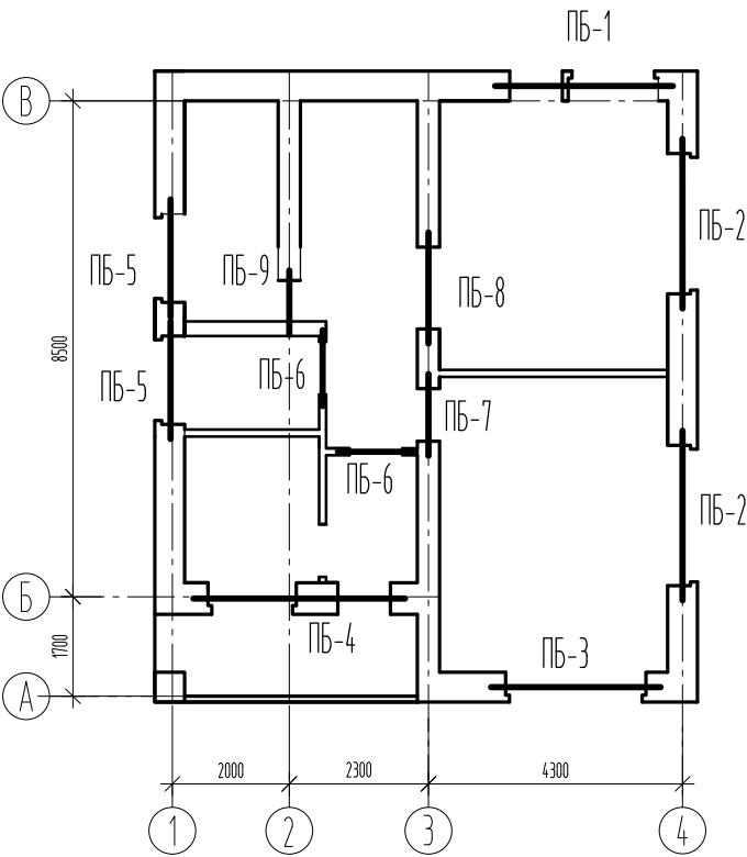
ПЛАН ПЕРЕМЫЧЕК 1 ЭТАЖА
