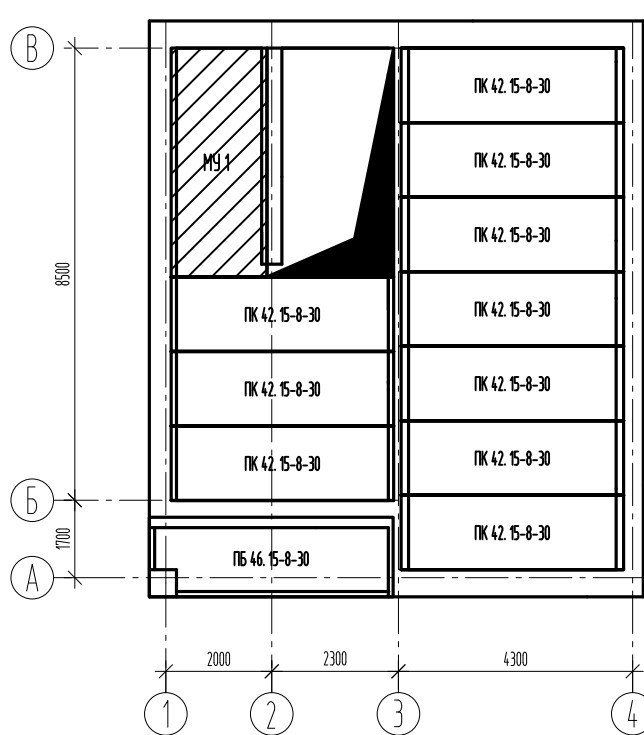
ПЛАН ПЕРЕКРЫТИЙ
