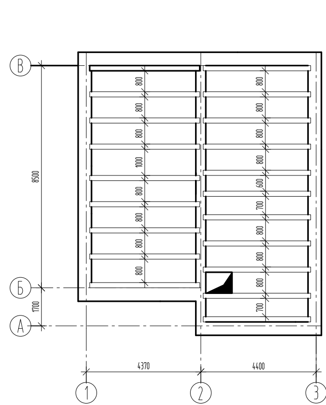
ПЛАН ДЕРЕВЯННЫХ ПЕРЕКРЫТИЙ
