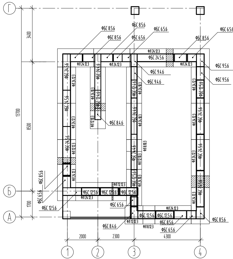
ПЛАН ФУНДАМЕНТА
