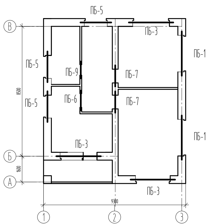
ПЛАН ПЕРЕМЫЧЕК 2 ЭТАЖА
