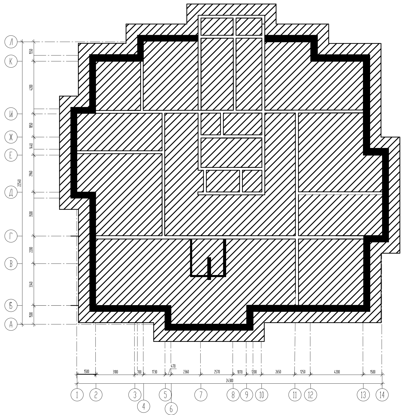
ПЛАН ФУНДАМЕНТА
