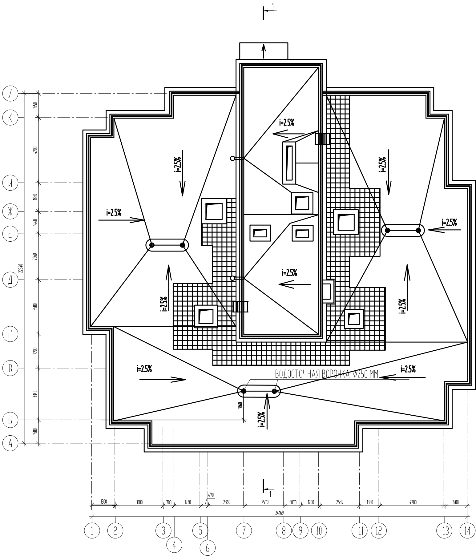
ПЛАН КРОВЛИ
