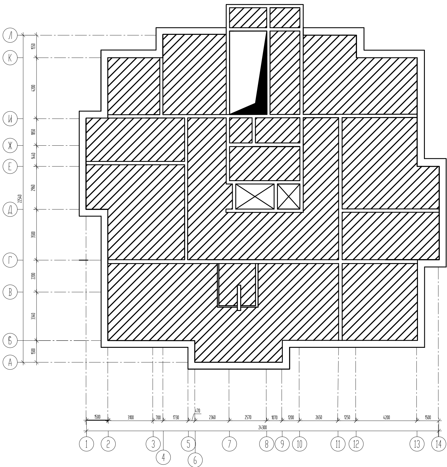
ПЛАН ПЕРЕКРЫТИЙ И ПОКРЫТИЯ
