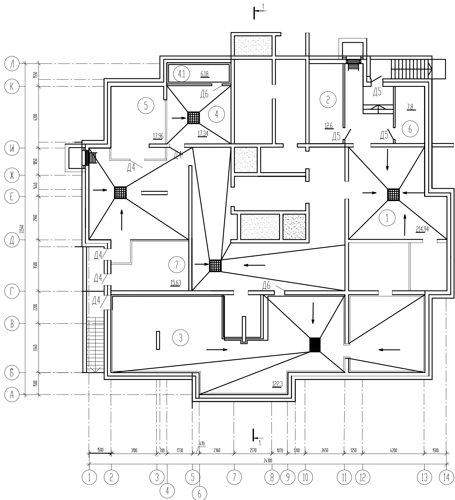
ПЛАН ПОДВАЛА
