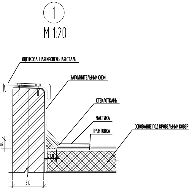
УЗЕЛ ПРИМЫКАНИЯ ПРИМЫКАНИЯ КРОВЛИ К ПАРАПЕТУ
