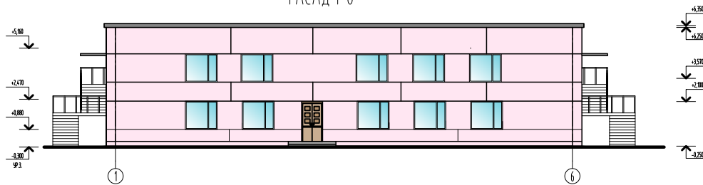
ФАСАД 1-6
