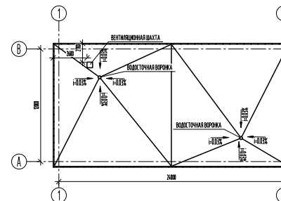
ПЛАН КРОВЛИ
