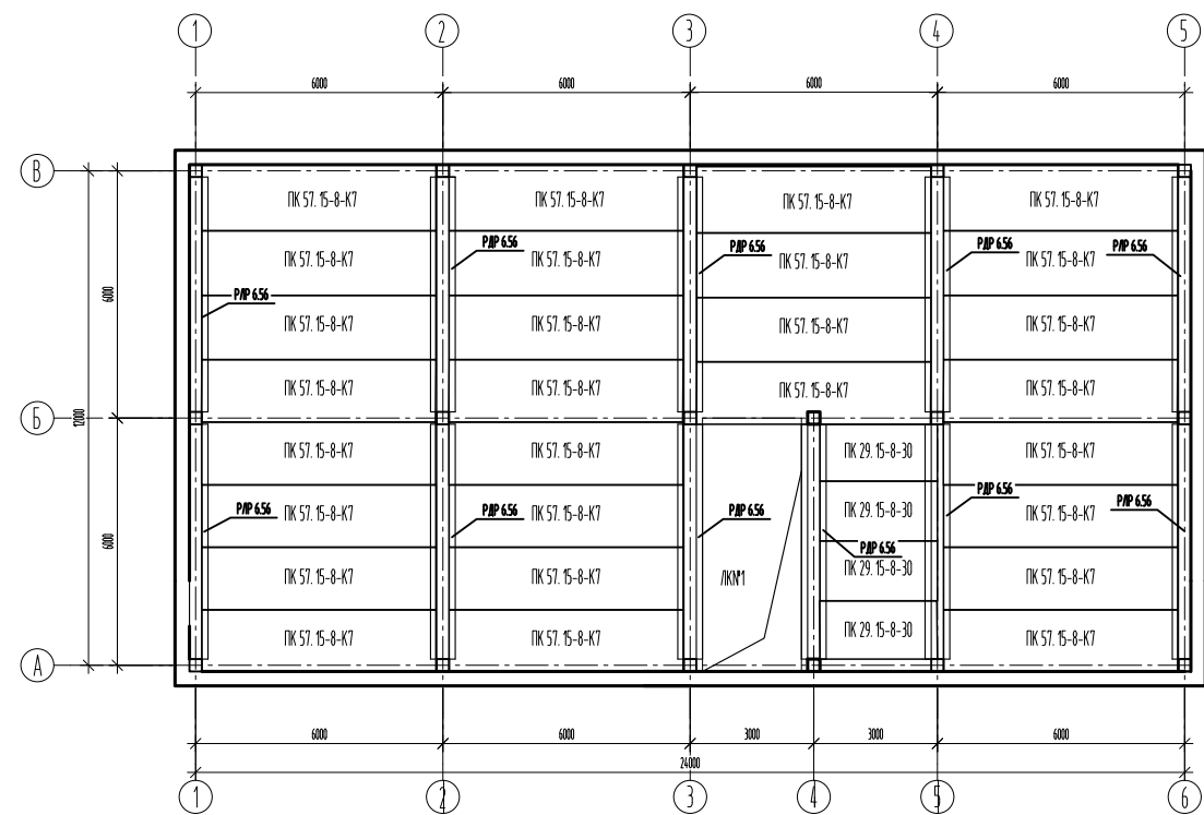
ПЛАН ПЕРЕКРЫТИЙ
