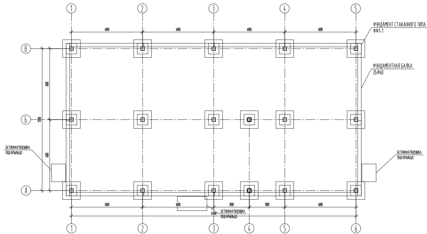
ПЛАН ФУНДАМЕНТА
