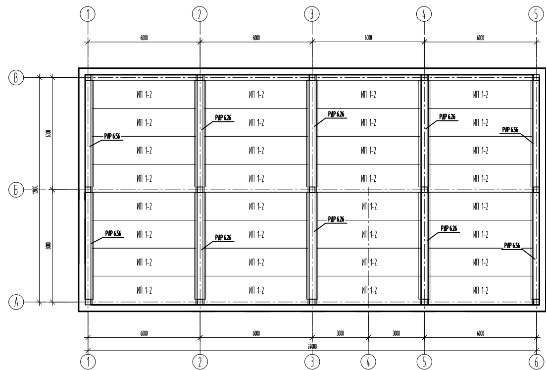
ПЛАН ПОКРЫТИЯ
