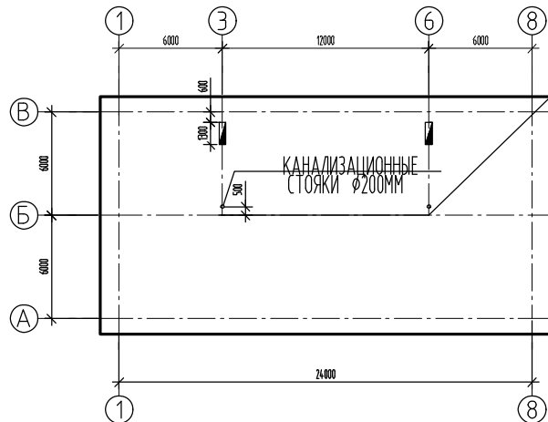
ПЛАН КРЫШИ
