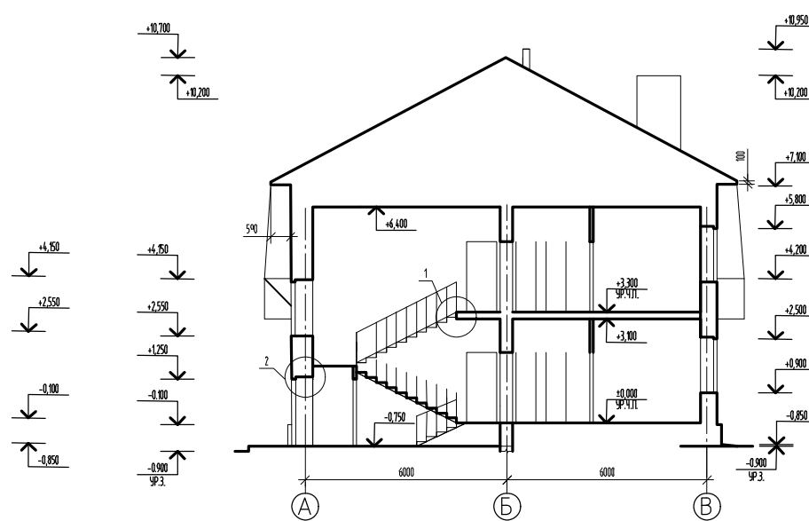
РАЗРЕЗ 1-1
