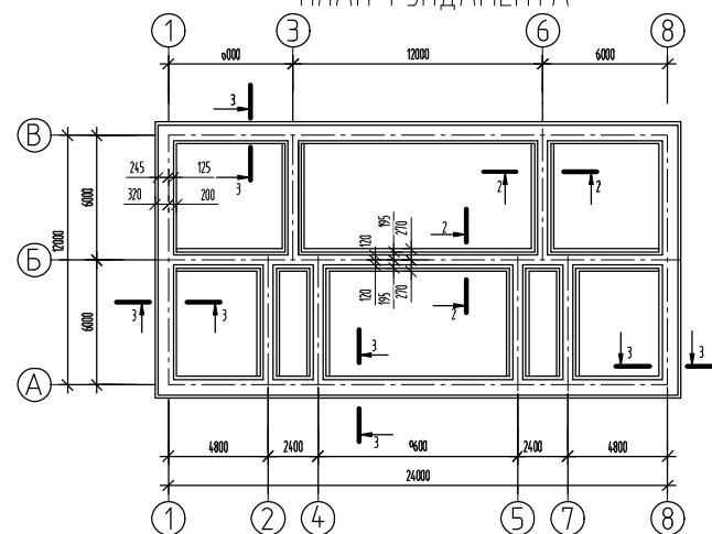
ПЛАН ФУНДАМЕНТА
