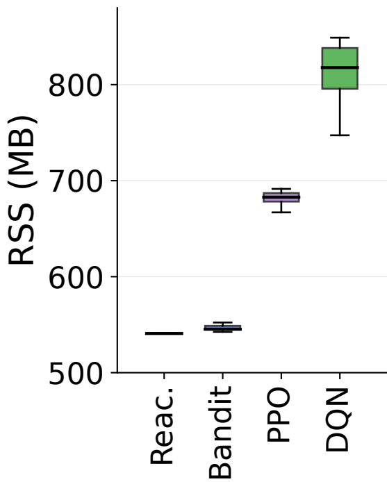
RSS
