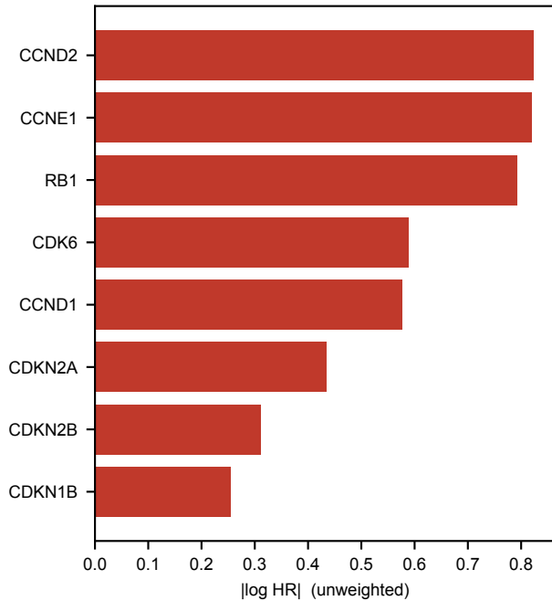
Cell_Cycle_zsum
