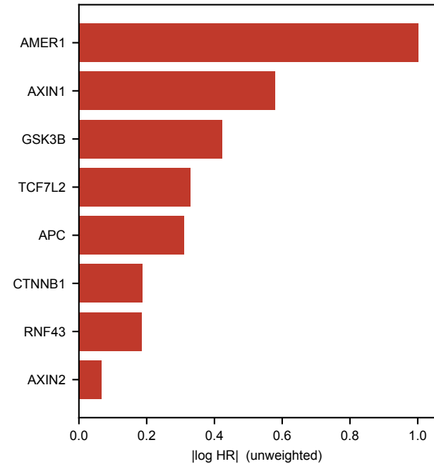
WNT_zsum
