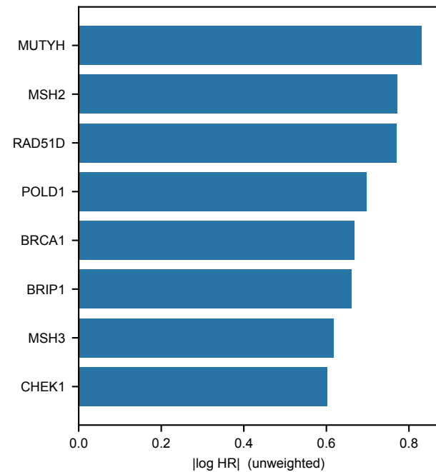
DDR_zsum
