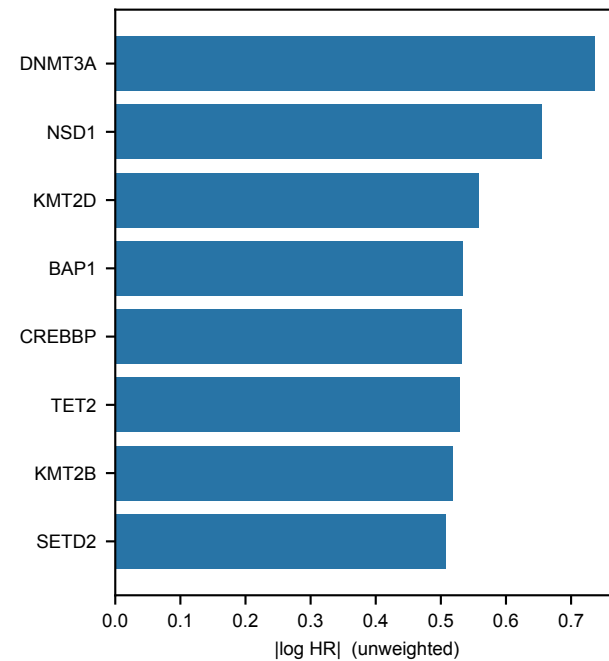
Chromatin_any_rate
