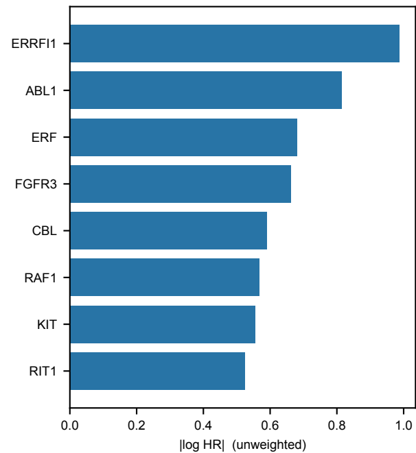
RTK_RAS_any_rate
