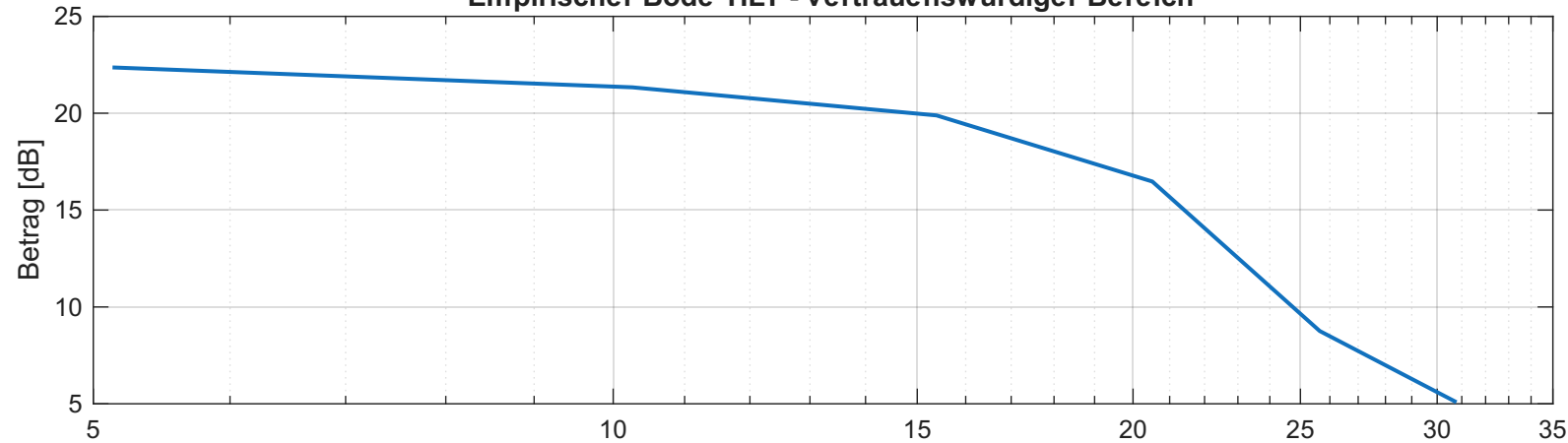
Empirischer Bode TILT - vertrauenswürdiger Bereich
