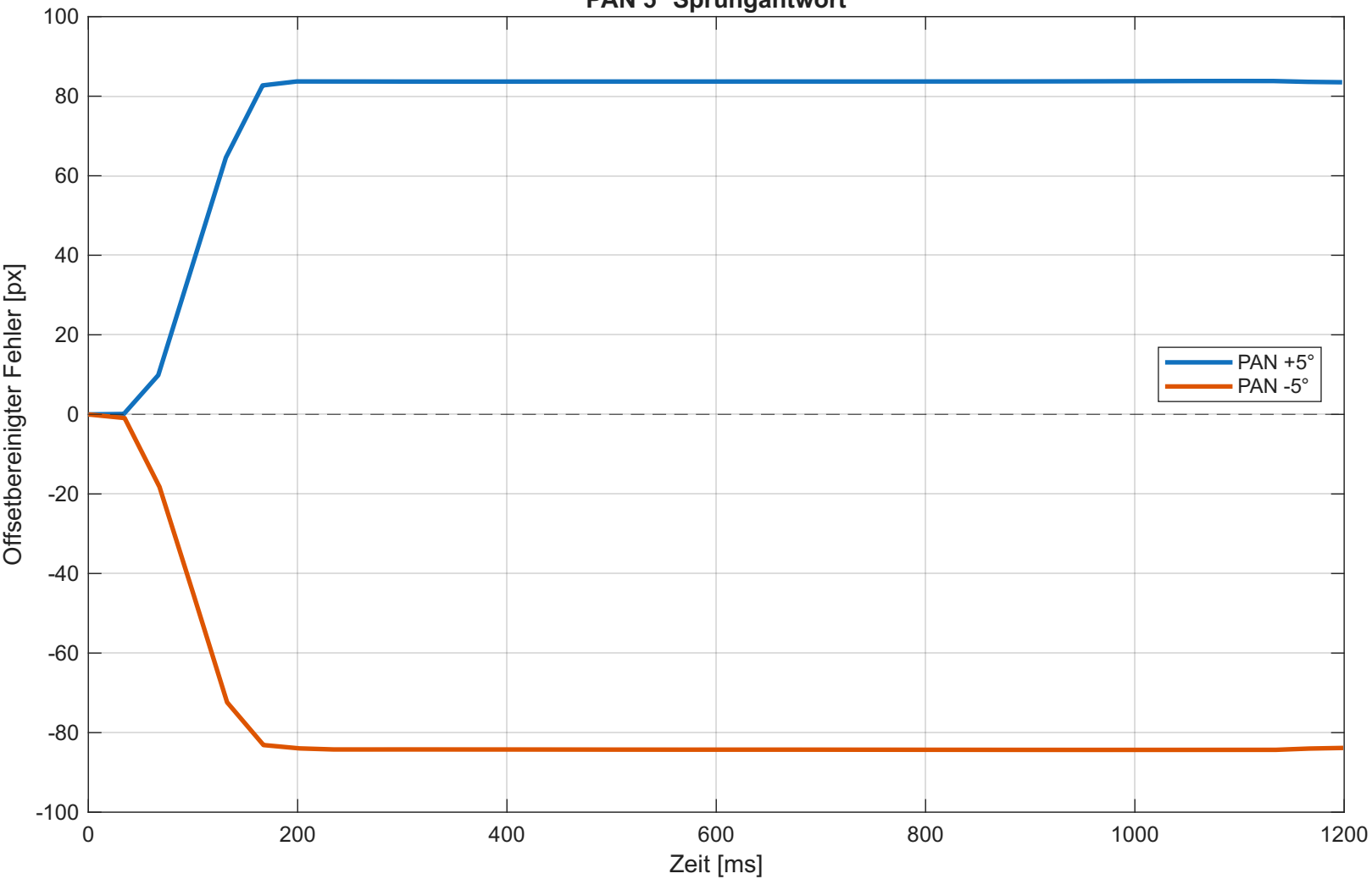
PAN 5° Sprungantwort
