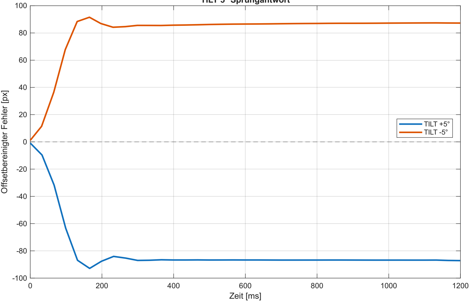
TILT 5° Sprungantwort
