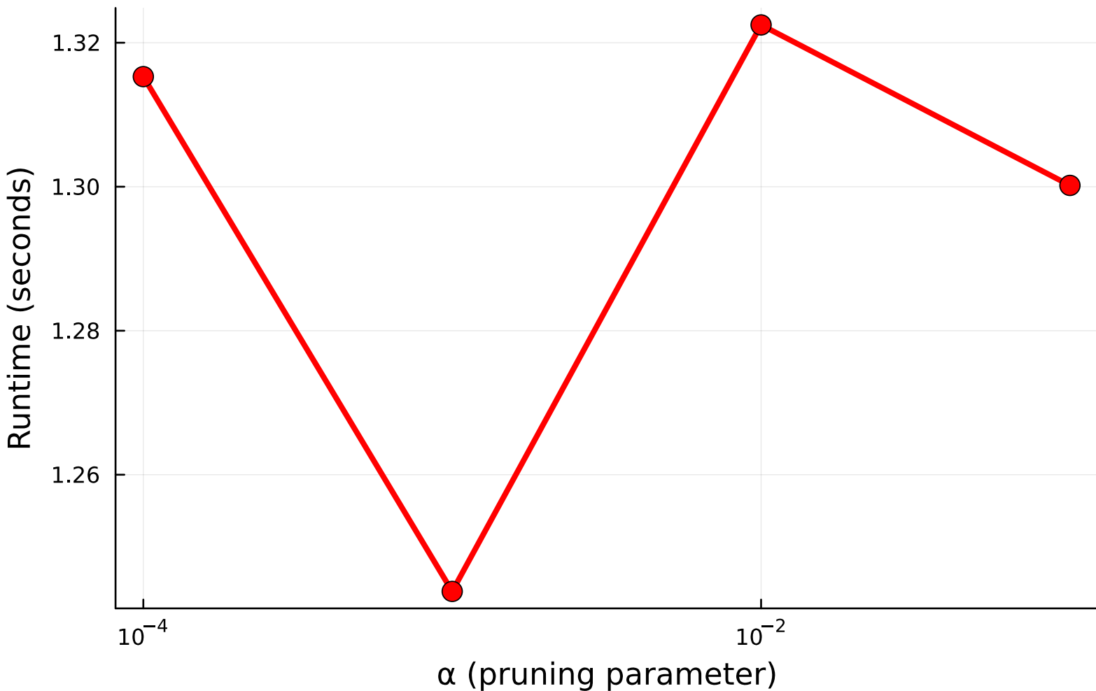
Runtime vs Alpha Parameter (N=16)
