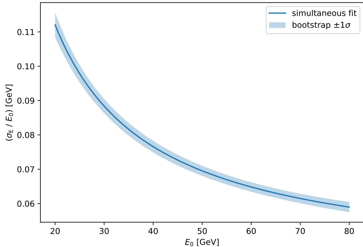
(\sigma_E / E_0) vs E_0
