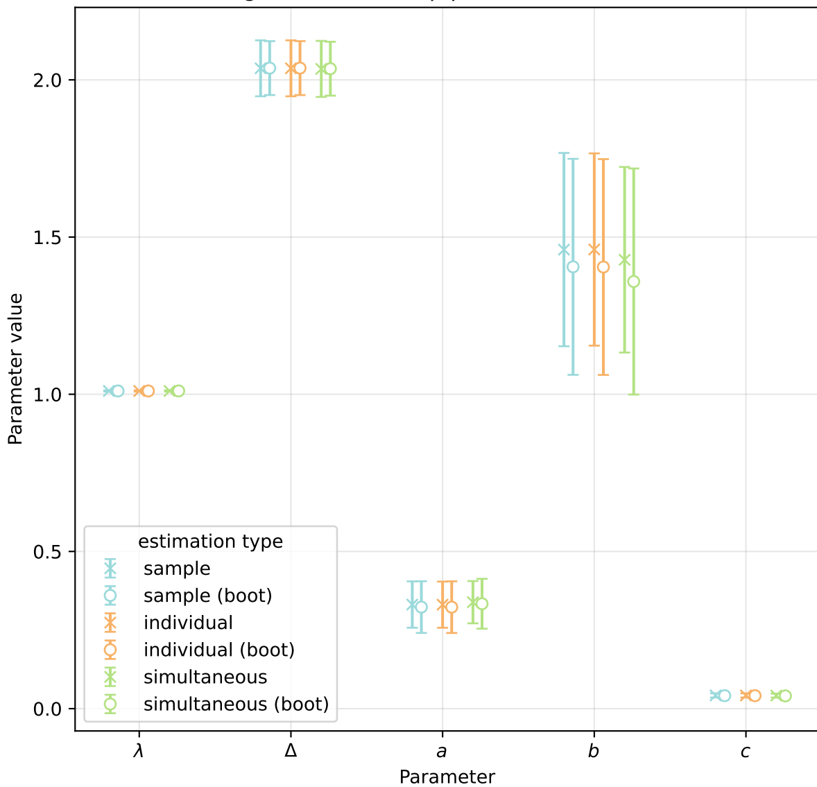
Original vs bootstrap parameter estimates
