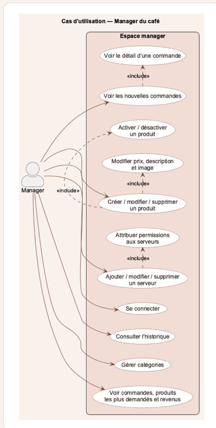
Figure 2 – Cas d'utilisation du manager.
