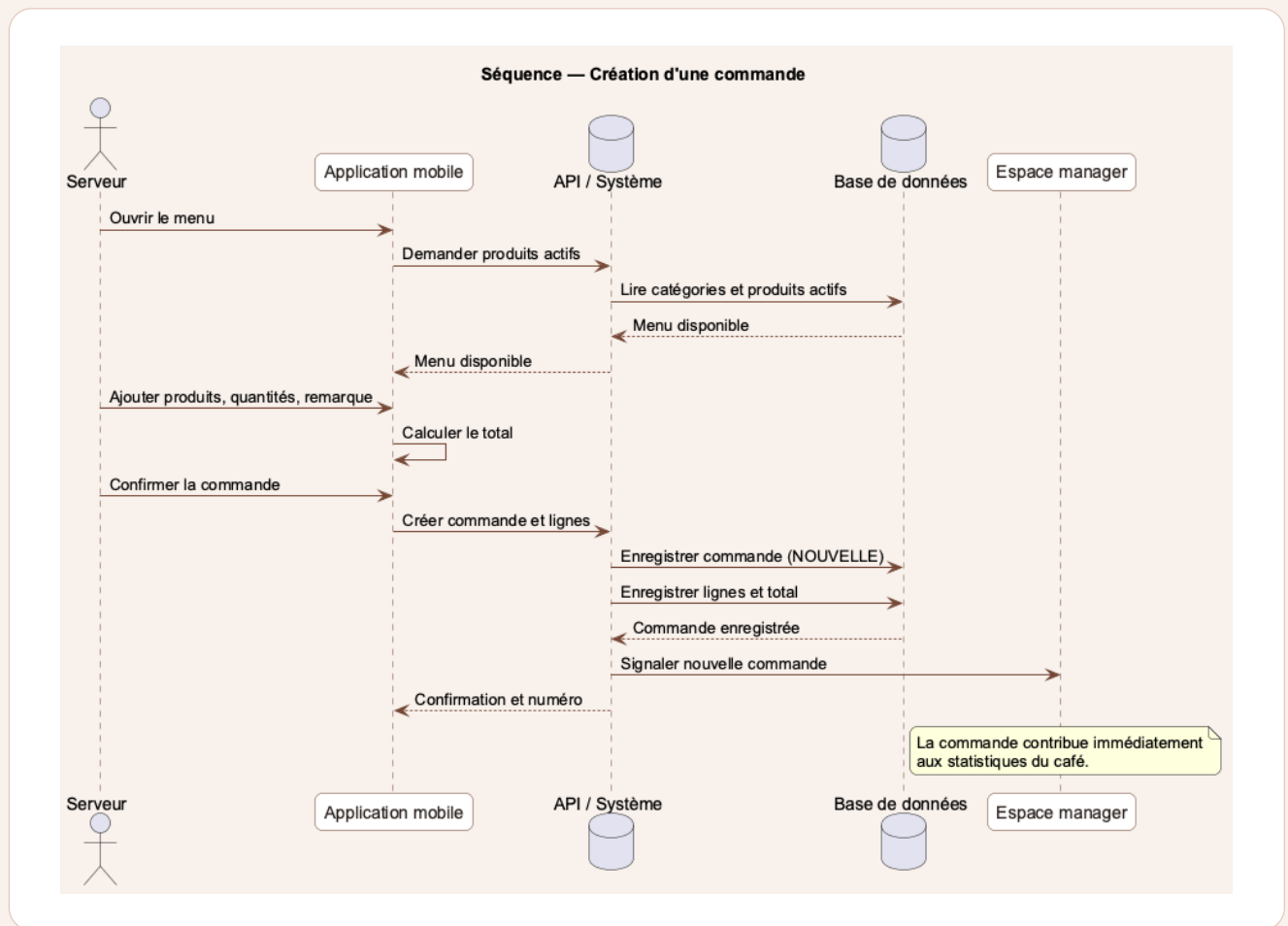
Figure 8 – Diagramme de séquence de création d'une commande.
