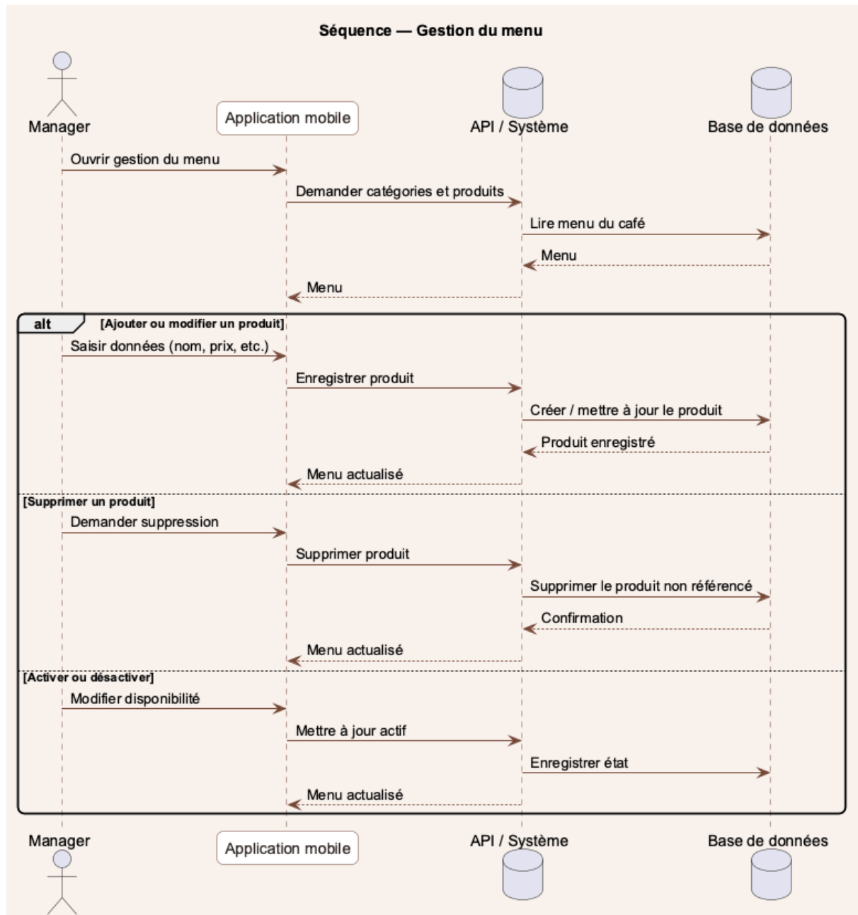
Figure 9 – Diagramme de séquence de gestion du menu.
