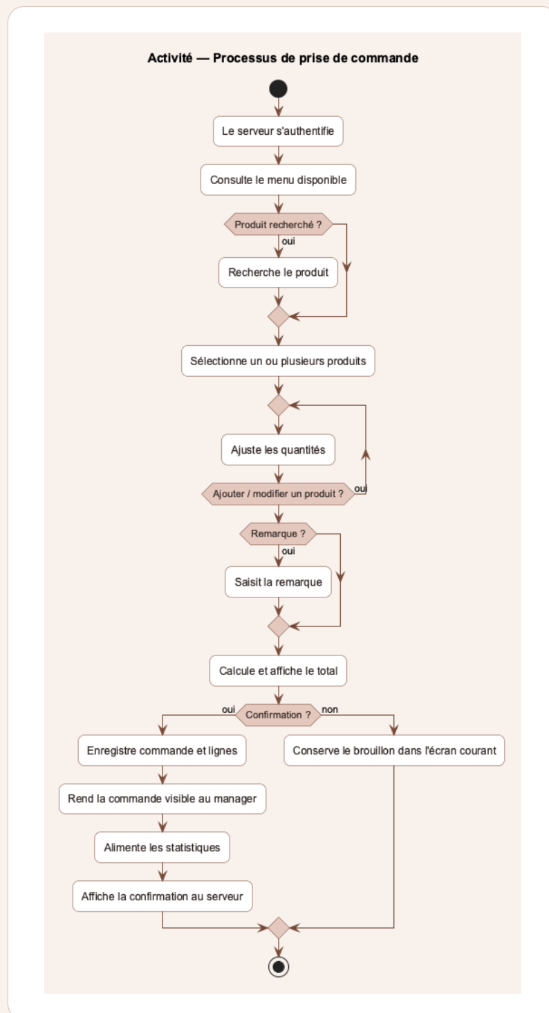
Figure 11 – Diagramme d'activité du processus de commande.
