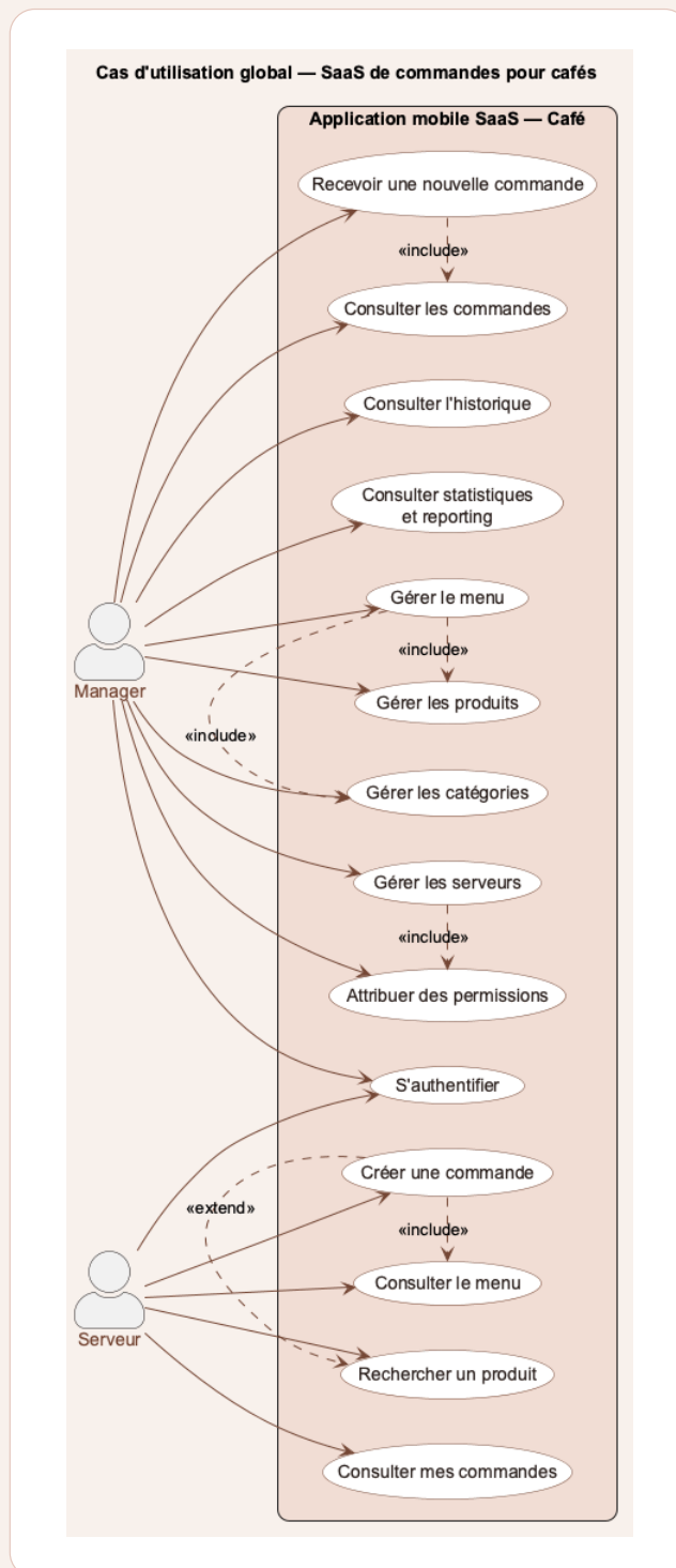
Figure 1 – Diagramme de cas d'utilisation global.
