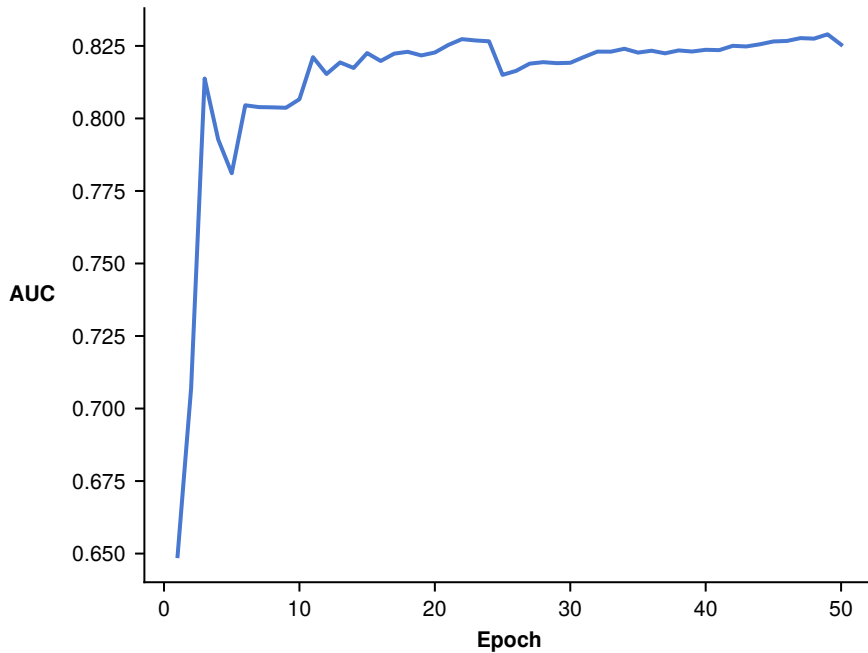
Val AUC
