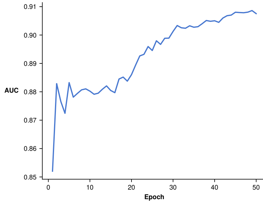
Val AUC
