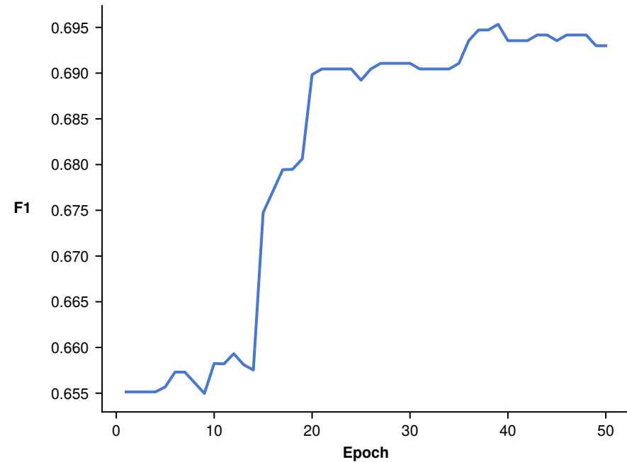
Val F1
