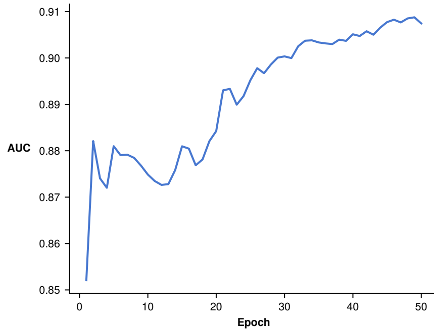
Val AUC
