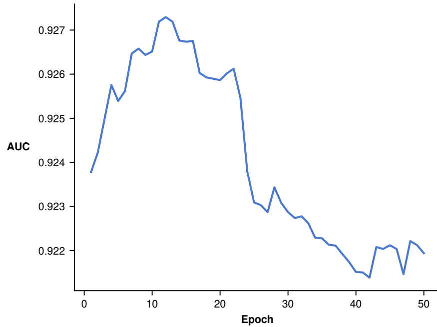
Val AUC
