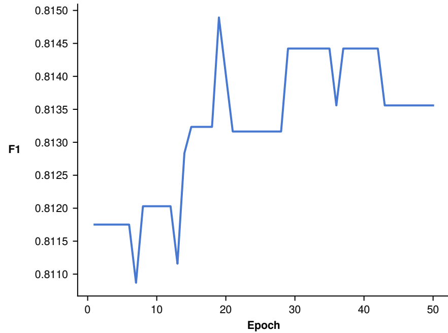
Val F1
