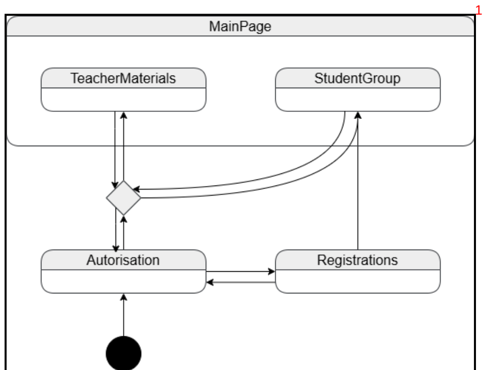
Рисунок 28 - диаграмма состояний системы при работе неизвестного пользователя
