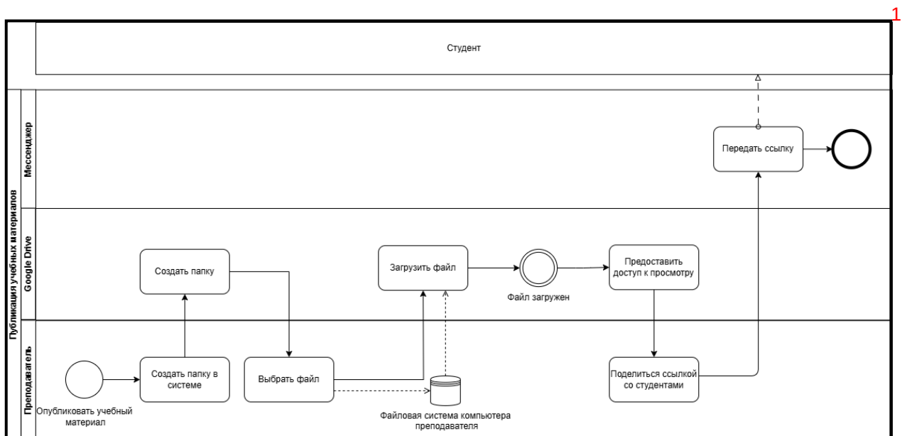
Рисунок 6 – AS-IS Схема публикации учебных материалов в интернет-среде
