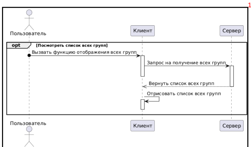
Рисунок 21 - диаграмма последовательности прецедента “Посмотреть список групп”
