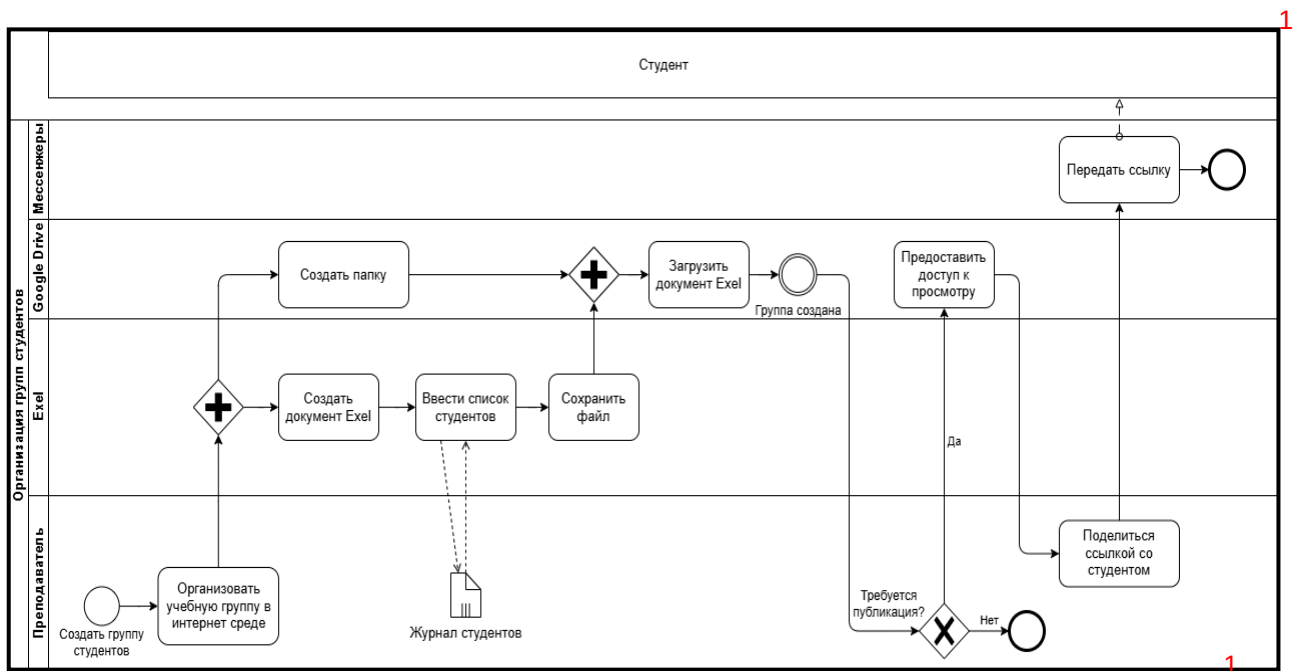
Рисунок 2 – AS-IS Схема организации групп студентов в интернет-среде
