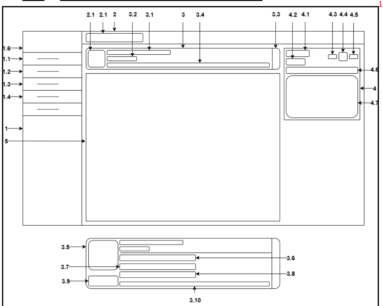
Рисунок 32 - Проект интерфейса основных элементов страницы 1
