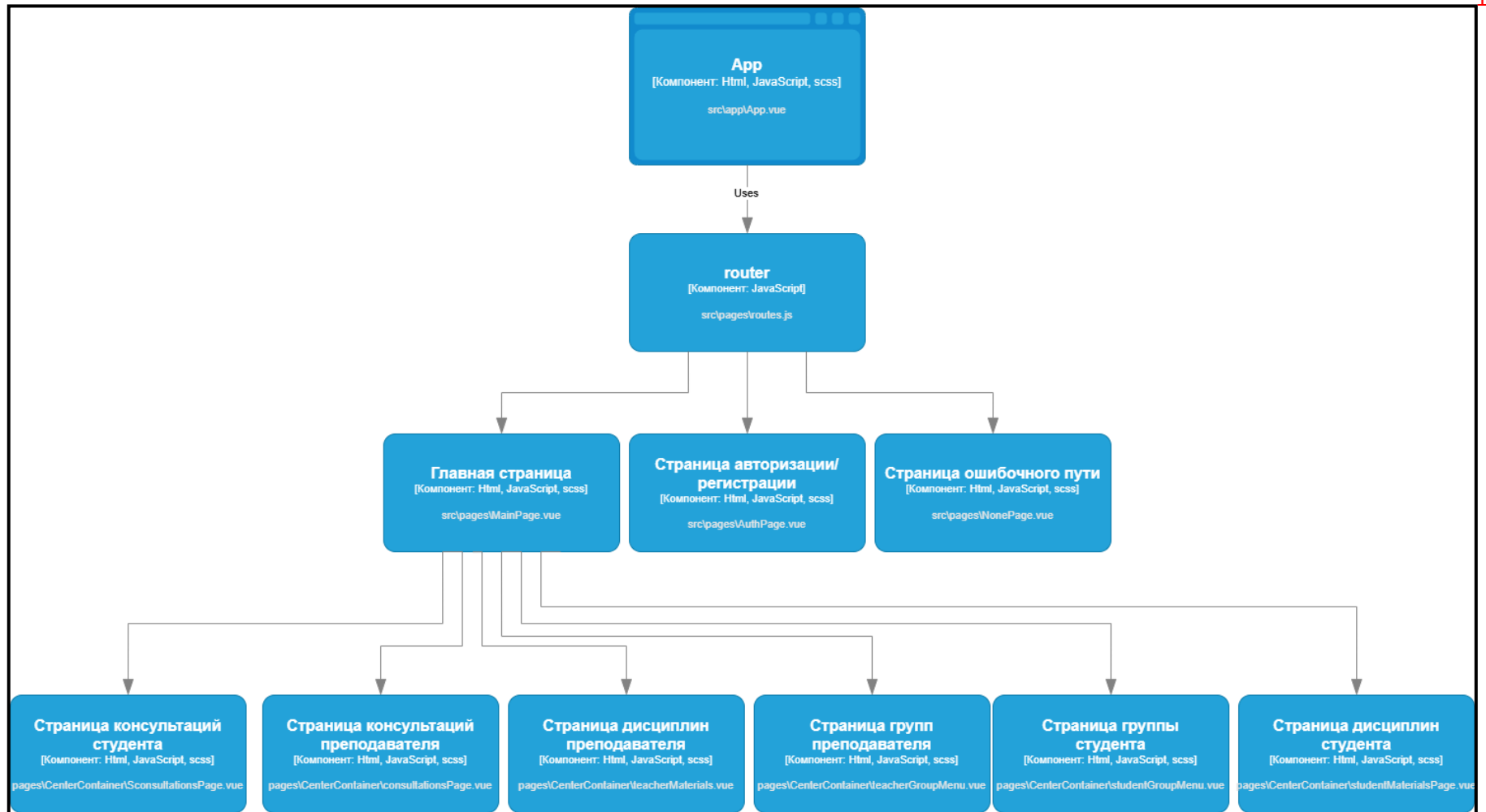
Рисунок Е.1 - UML диаграмма страниц приложения 1
