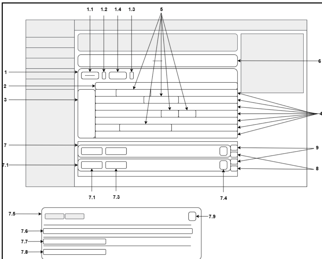
Рисунок 37 - Проект интерфейса страницы консультаций преподавателя
