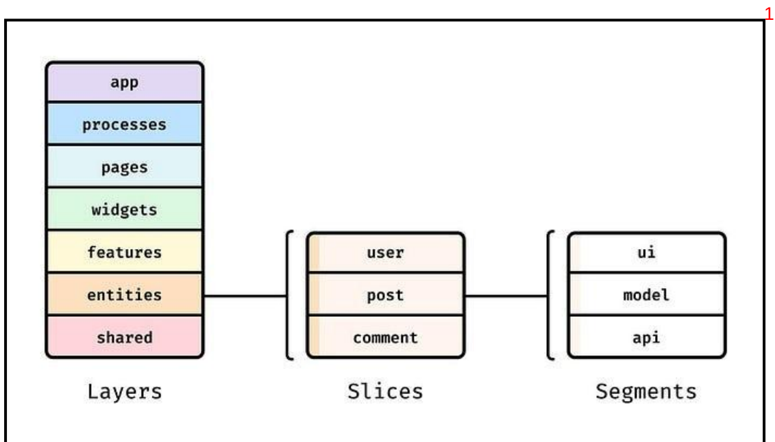
Рисунок 38 – Пример архитектуры FSD
