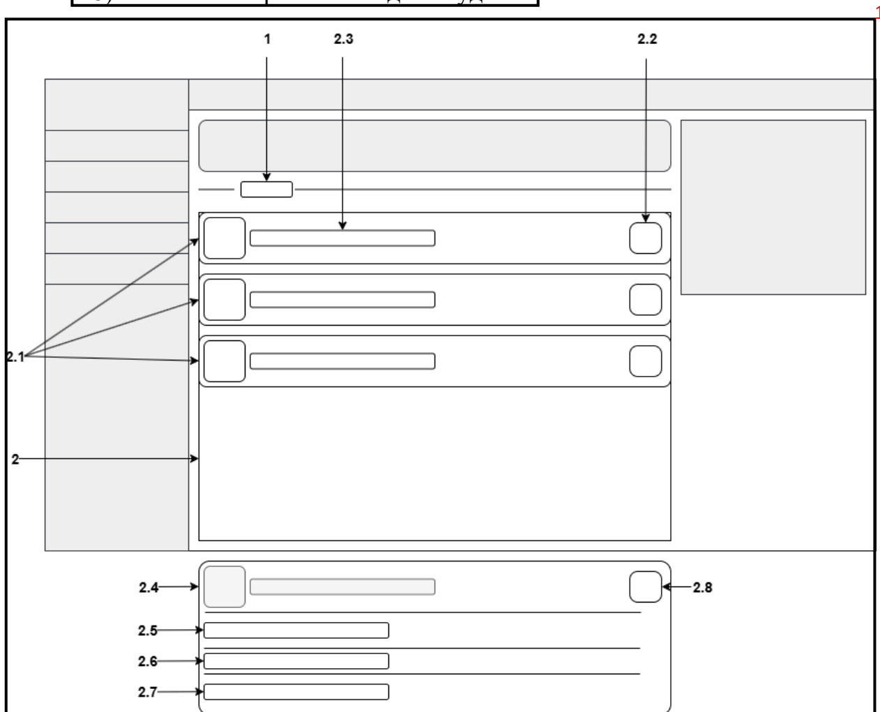
Рисунок 35 - Проект интерфейса страницы группы студента 1
