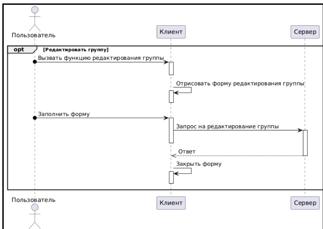
Рисунок 24 - диаграмма последовательности прецедента “Редактировать группу”
