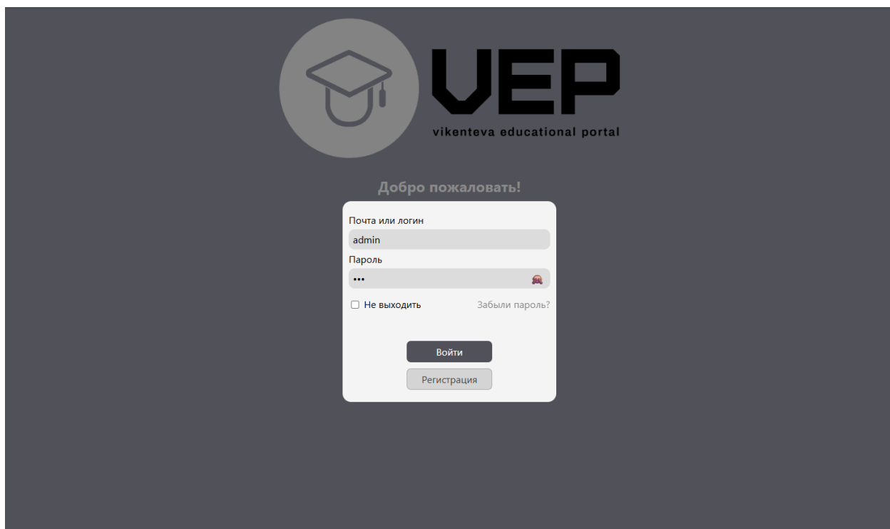
Рисунок 40 - страница авторизации 0.41
