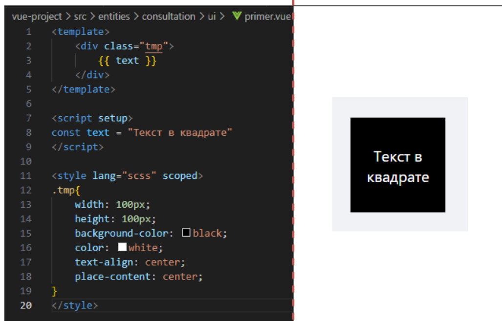
Рисунок 39 – Пример компонента vue
