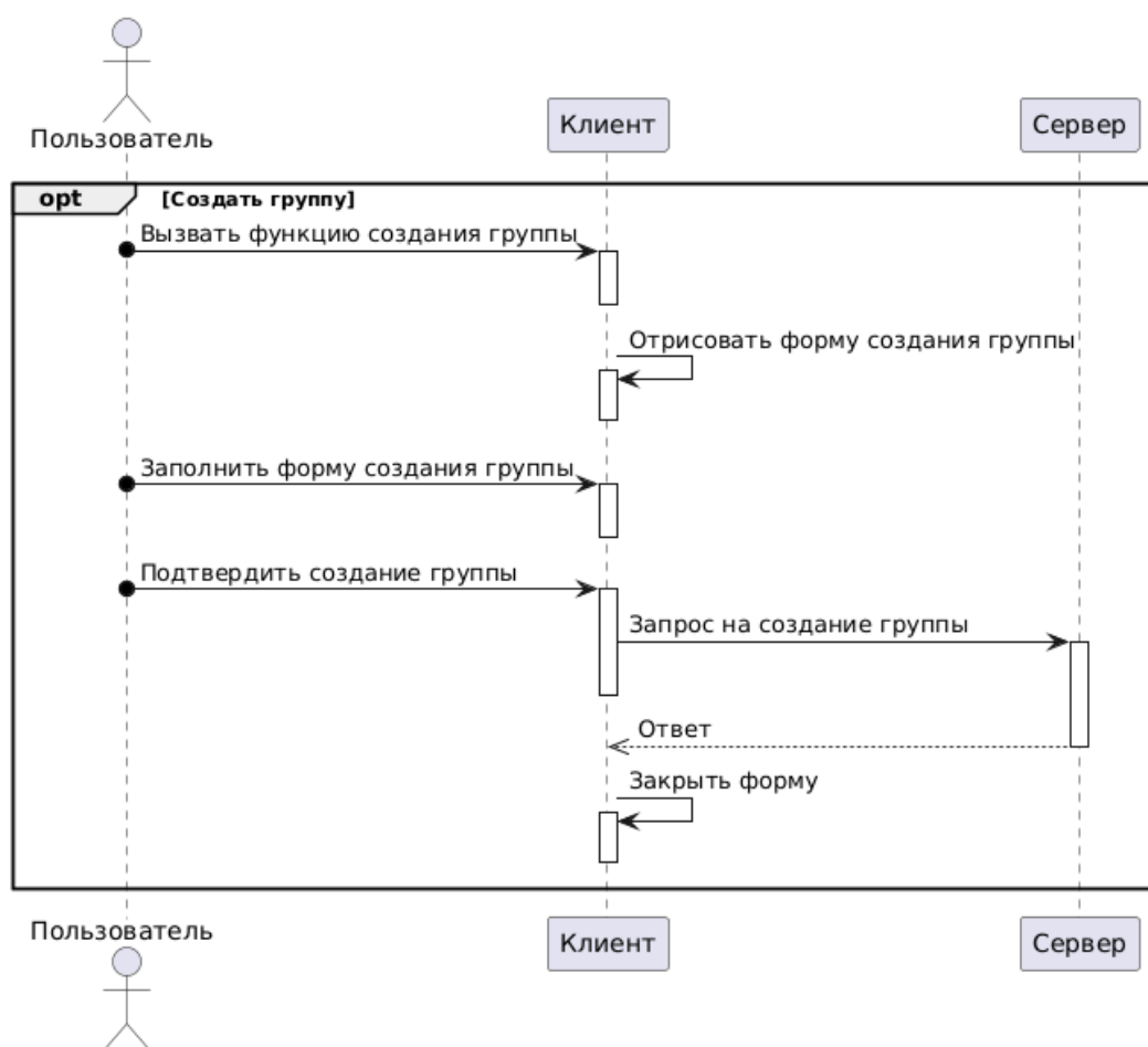
Рисунок 23 - диаграмма последовательности прецедента “Создать группу”
