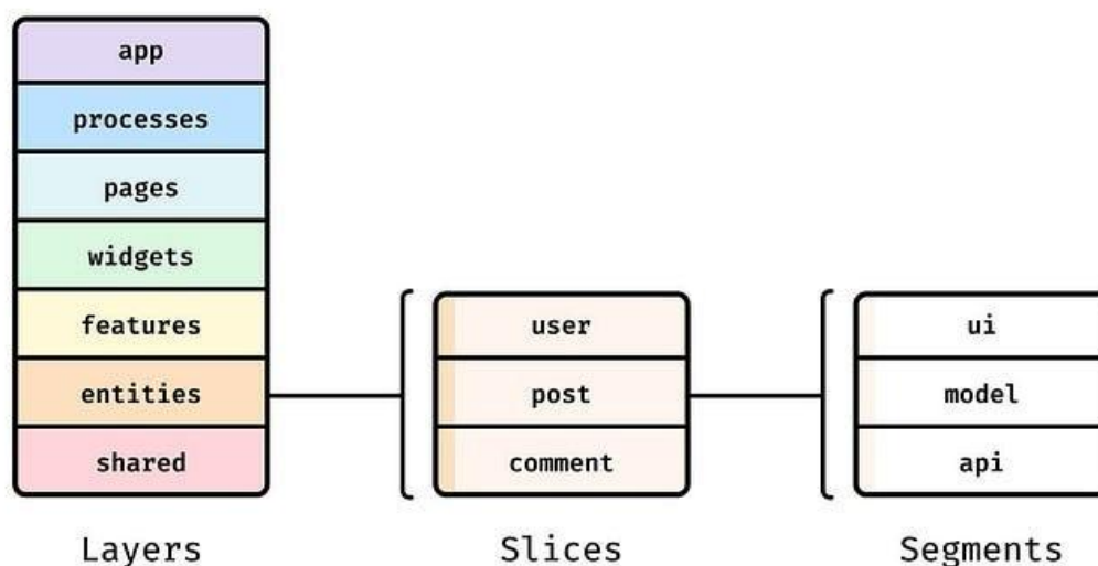
Рисунок 38 – Пример архитектуры FSD
