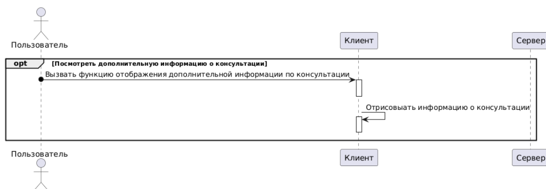
Рисунок 27 - диаграмма последовательности прецедента “Посмотреть дополнительную информацию о консультации”
