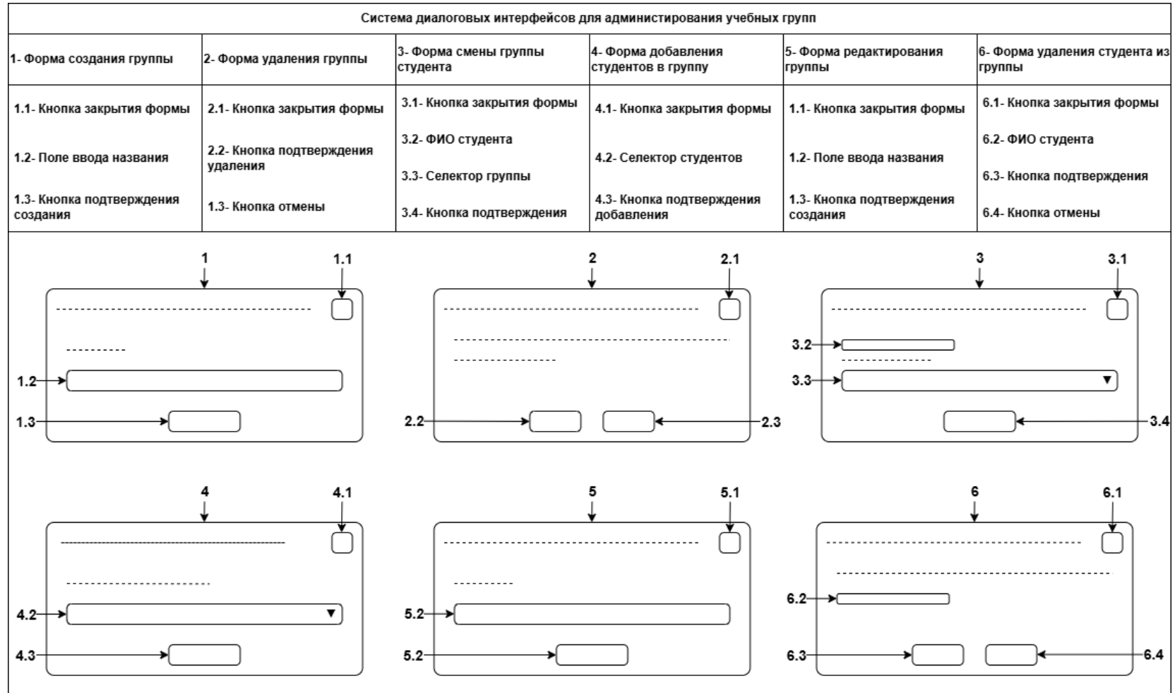
Рисунок А.1 - Проект интерфейсов диалоговых форм для администрирования групп
