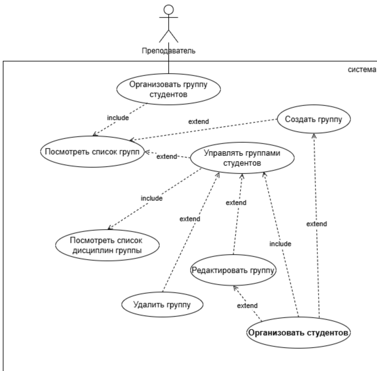
Рисунок 14 – Подробная диаграмма вариантов использования системы для прецедента “Организовать группу студентов”
