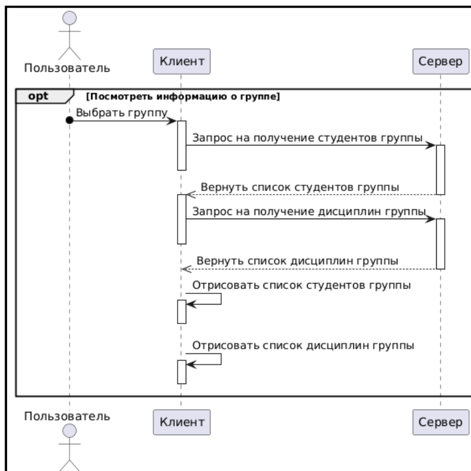
Рисунок 22 - диаграмма последовательности прецедента “Управлять группами студентов [посмотреть список дисциплин группы, посмотреть список студентов группы]”
