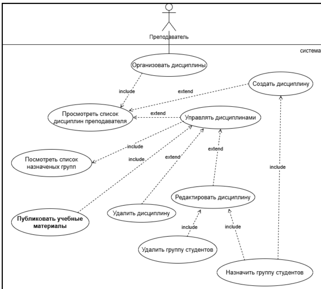
Рисунок 16- Подробная диаграмма вариантов использования системы для прецедента “организовать дисциплины”
