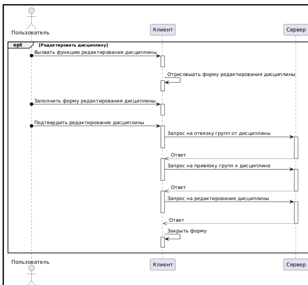
Рисунок 26 - диаграмма последовательности прецедента “Редактировать дисциплину”
