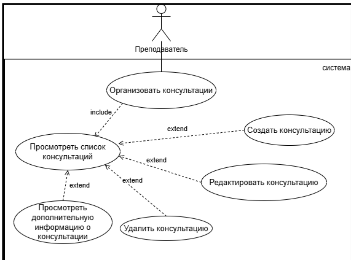
Рисунок 17- Подробная диаграмма вариантов использования системы для прецедента “организовать консультации”
