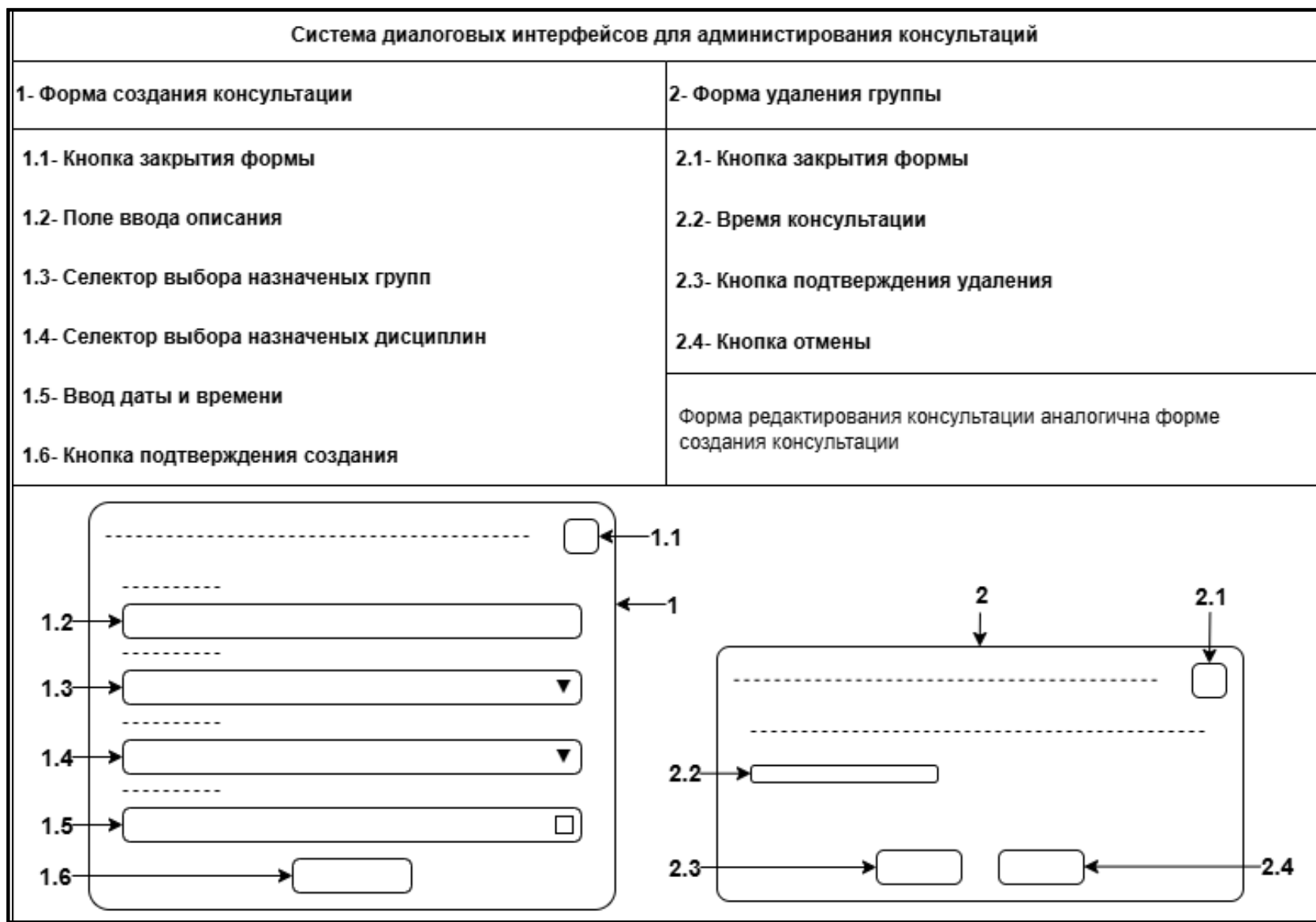
Рисунок А.3 - Проект интерфейсов диалоговых форм для администрирования консультаций
