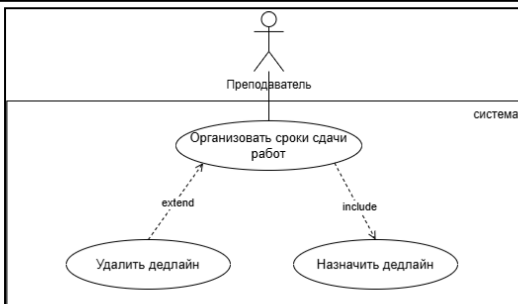
Рисунок 19- Подробная диаграмма вариантов использования системы для прецедента “Организовать сроки сдачи работ”
