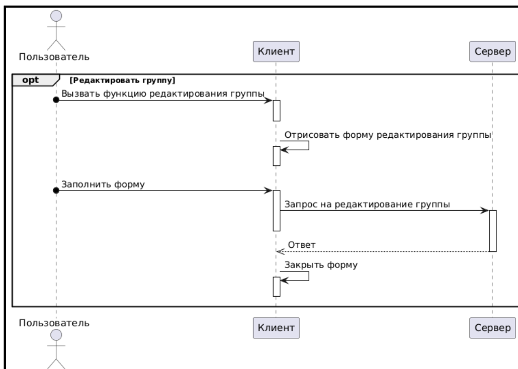
Рисунок 24 - диаграмма последовательности прецедента “Редактировать группу”
