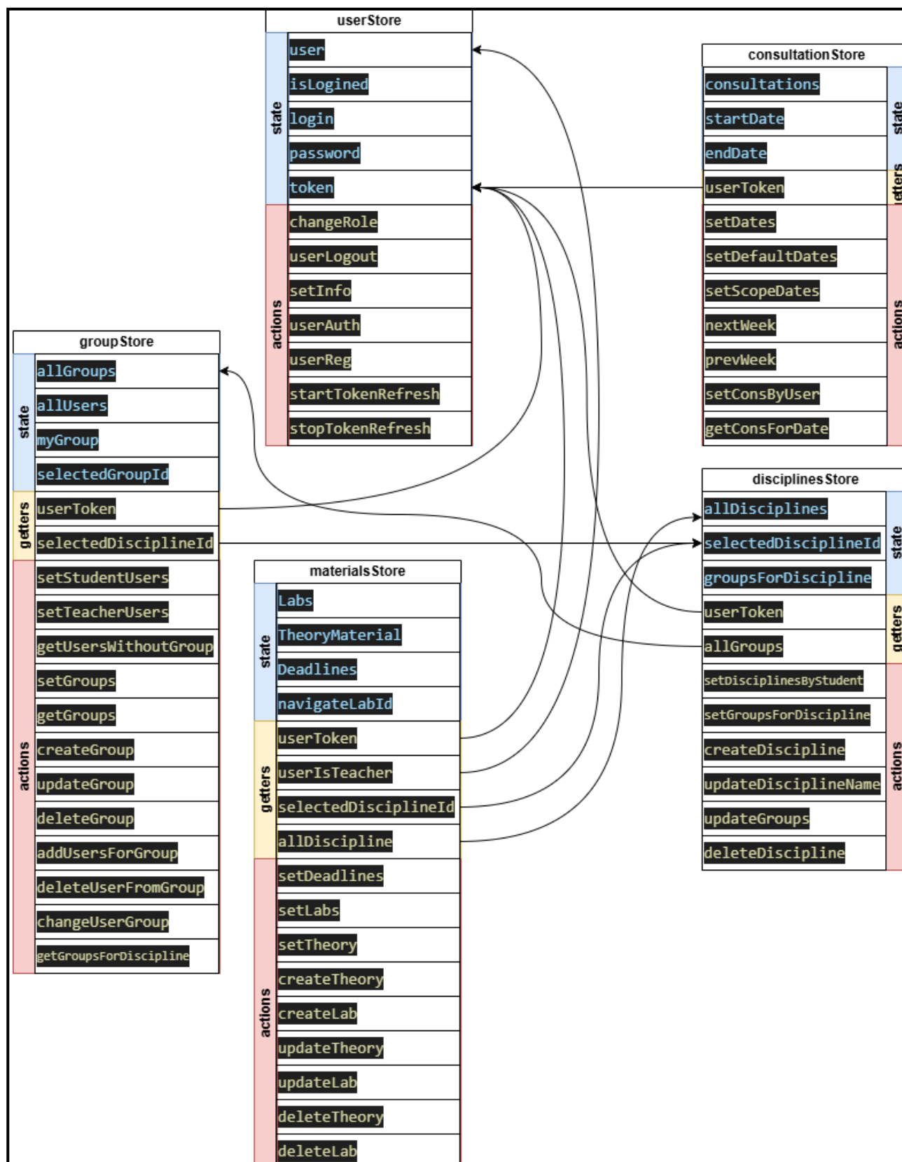
Рисунок Д.1 - диаграмма модульных хранилищ и их связей
