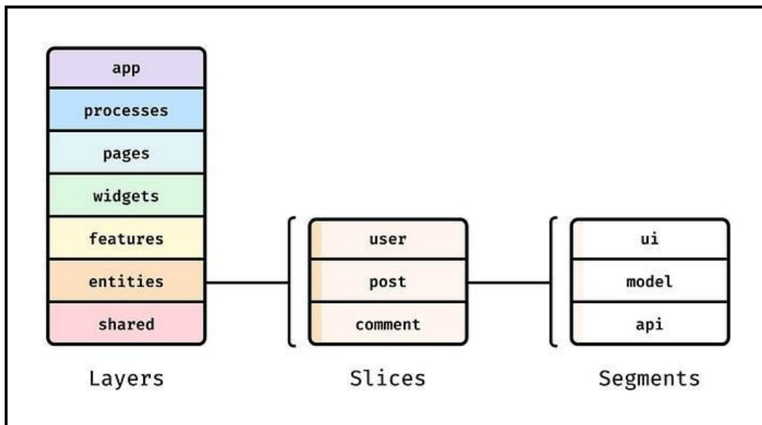
Рисунок 38 – Пример архитектуры FSD
