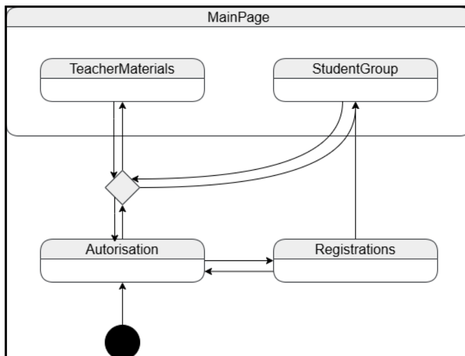
Рисунок 28 - диаграмма состояний системы при работе неизвестного пользователя
