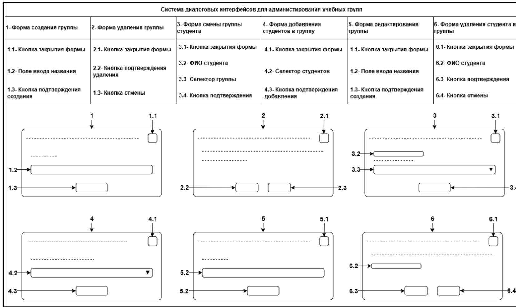
Рисунок А.1 - Проект интерфейсов диалоговых форм для администрирования групп
