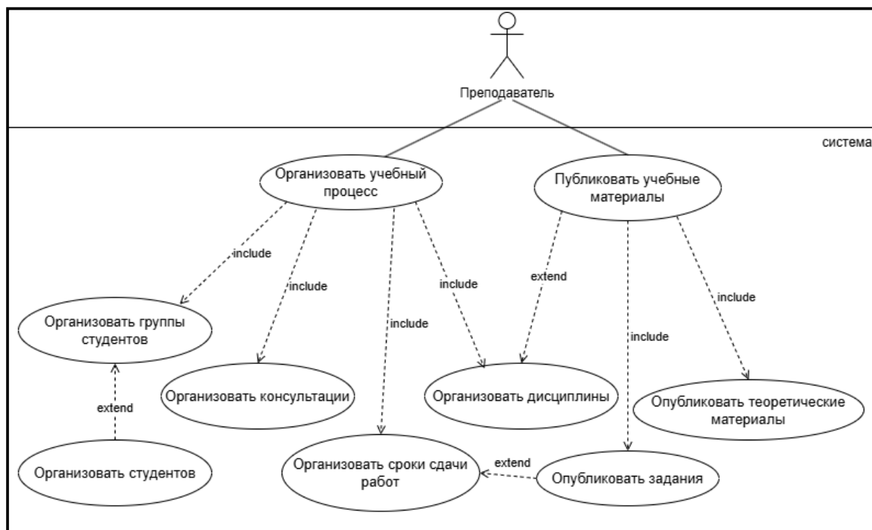
Рисунок 13 – Диаграмма вариантов использования системы для преподавателя
