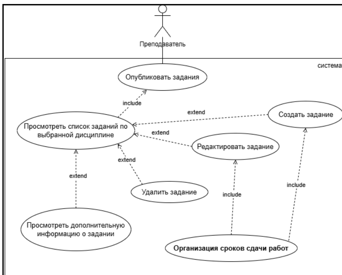
Рисунок 18- Подробная диаграмма вариантов использования системы для прецедента “опубликовать задания”
