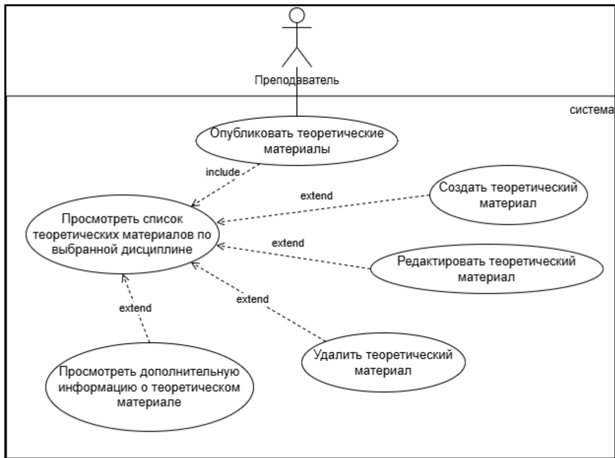
Рисунок 20- Подробная диаграмма вариантов использования системы для прецедента “Опубликовать теоретические материалы”
