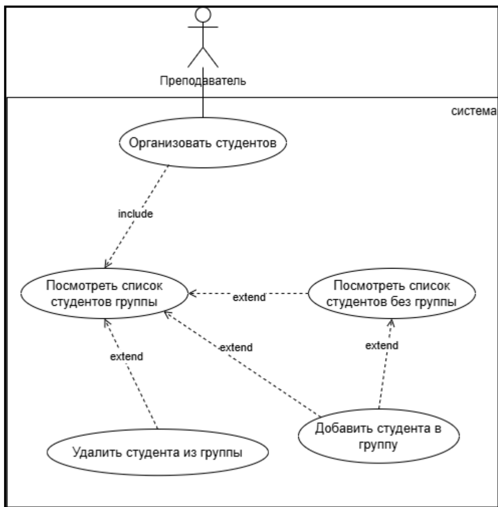
Рисунок 15 – Подробная диаграмма вариантов использования системы для прецедента “Организовать студентов”
