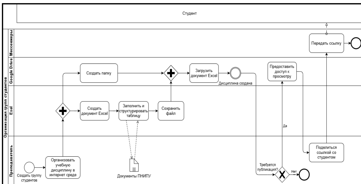
Рисунок 4 – AS-IS Схема организации дисциплины в интернет-среде
