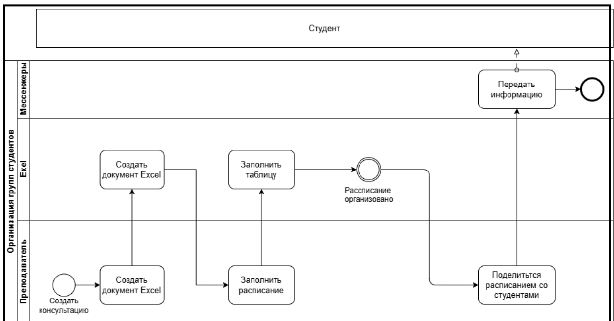
Рисунок 5 – AS-IS Схема организации консультаций и публикации расписания в интернет-среде
