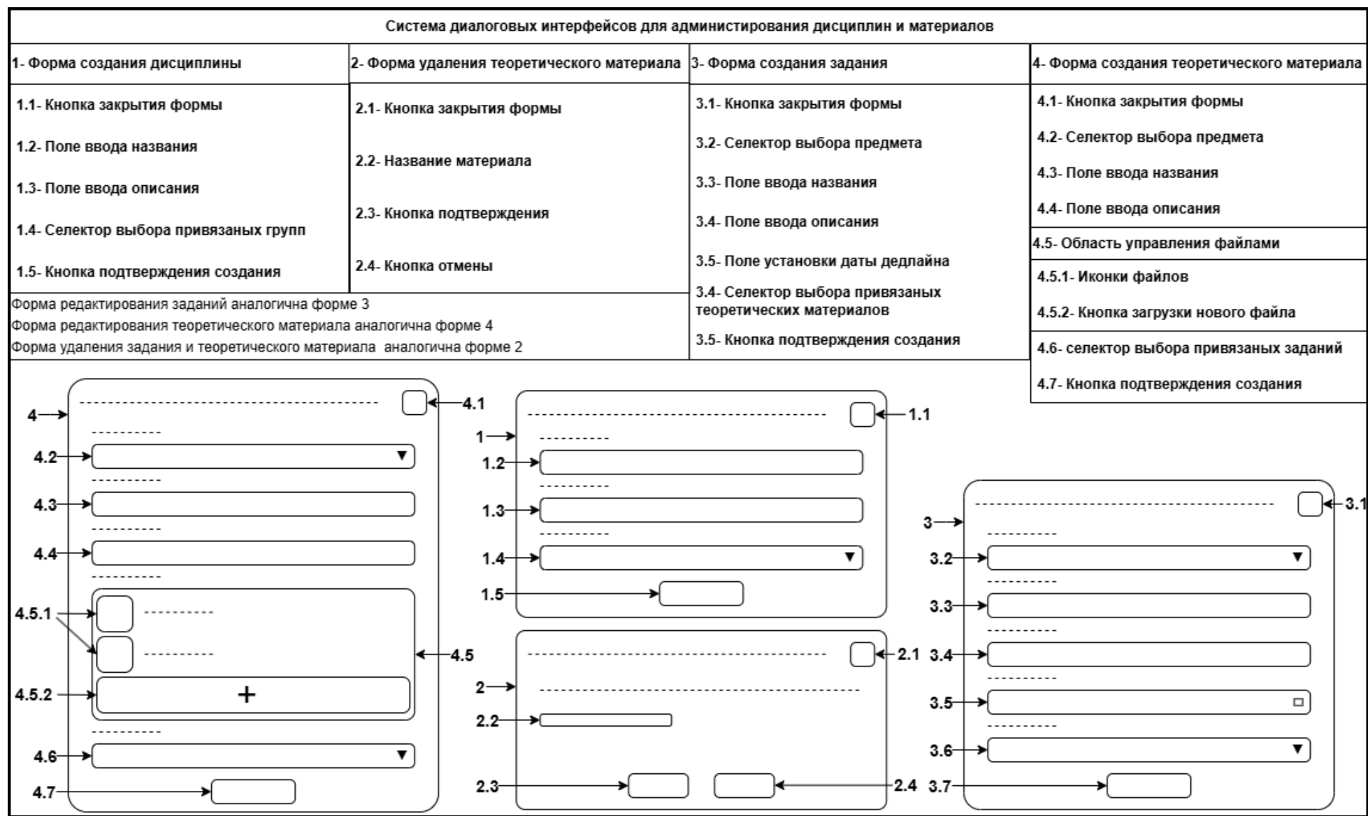
Рисунок А.2 - Проект интерфейсов диалоговых форм для администрирования дисциплин и материалов
