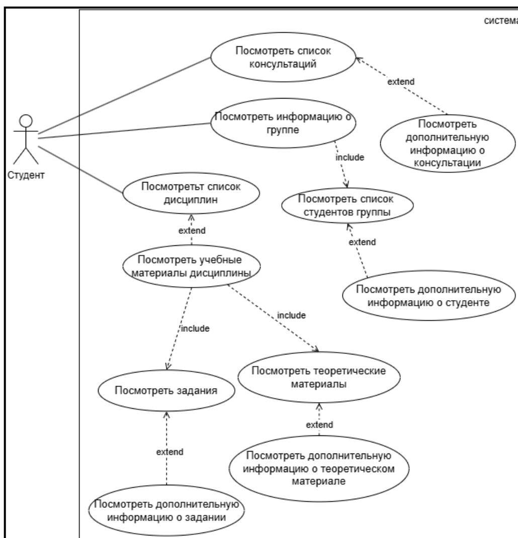
Рисунок 12 – Диаграмма вариантов использования системы для студента
