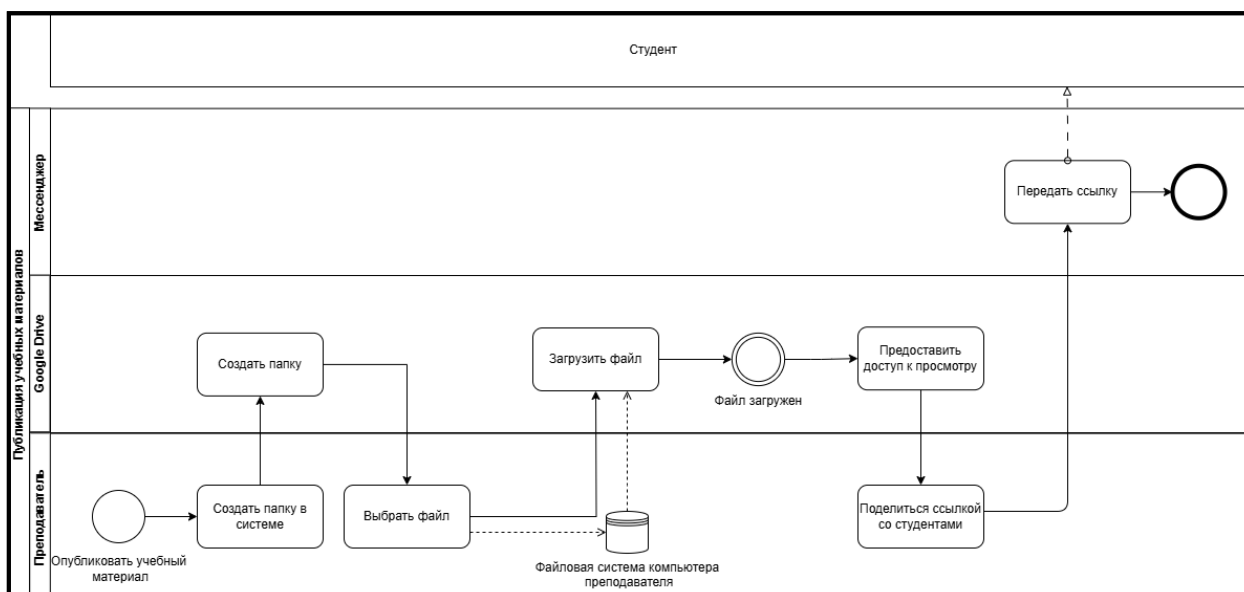
Рисунок 6 – AS-IS Схема публикации учебных материалов в интернет-среде
