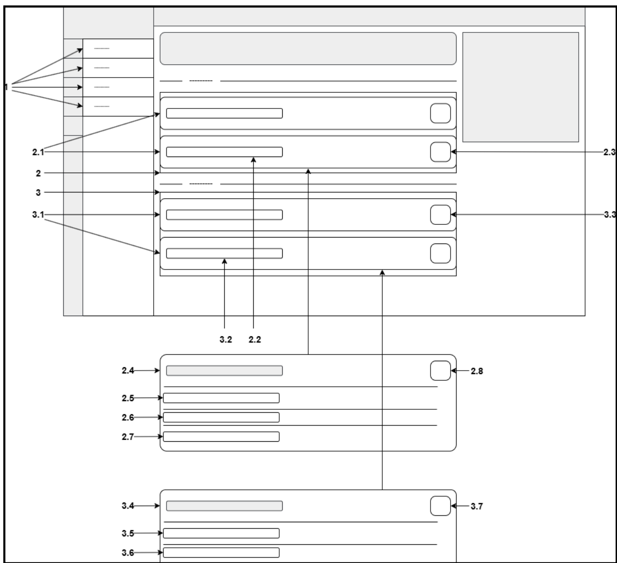
Рисунок 36 - Проект интерфейса страницы дисциплин и материалов студента
