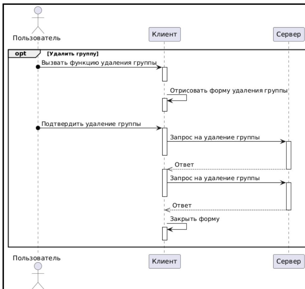
Рисунок 25 - диаграмма последовательности прецедента “удалить группу”
