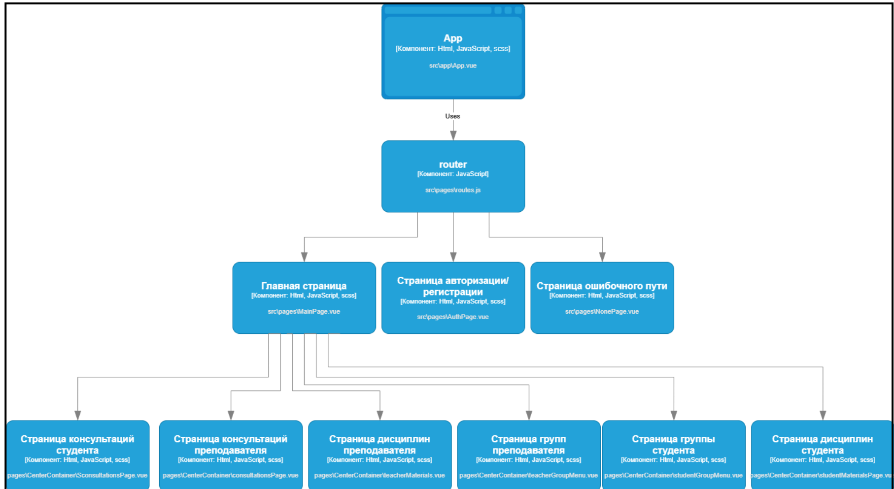
Рисунок Е.1 - UML диаграмма страниц приложения
