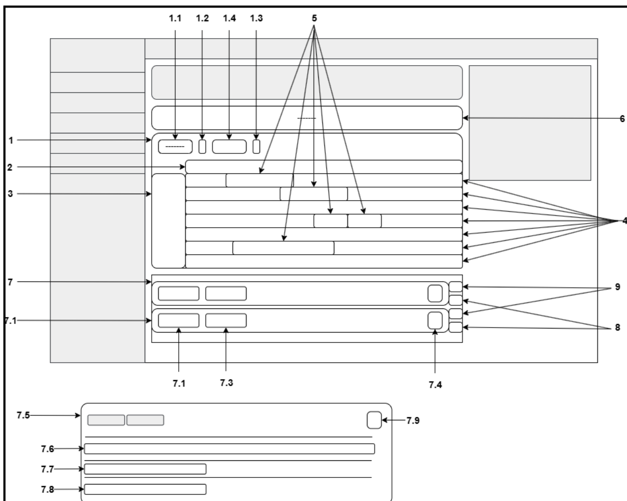
Рисунок 37 - Проект интерфейса страницы консультаций преподавателя
