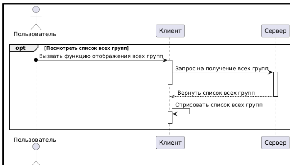
Рисунок 21 - диаграмма последовательности прецедента “Посмотреть список групп”
