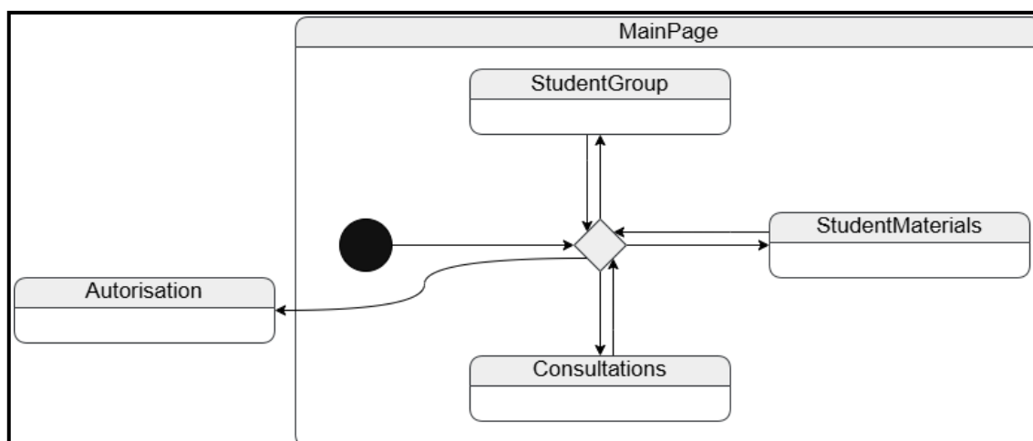
Рисунок 29 - диаграмма состояний системы при работе студента
