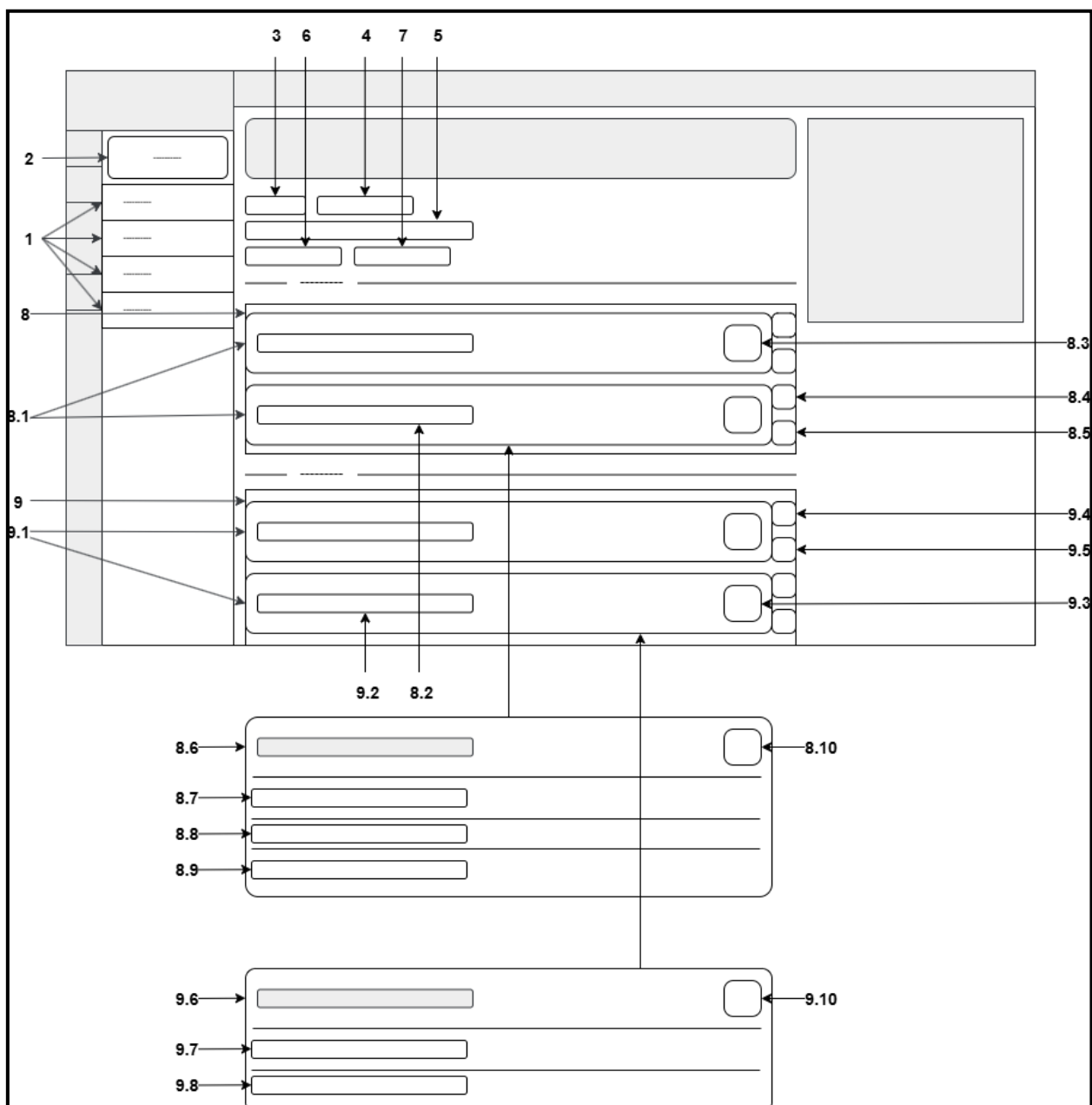
Рисунок 34 - Проект интерфейса страницы дисциплин и материалов преподавателя
