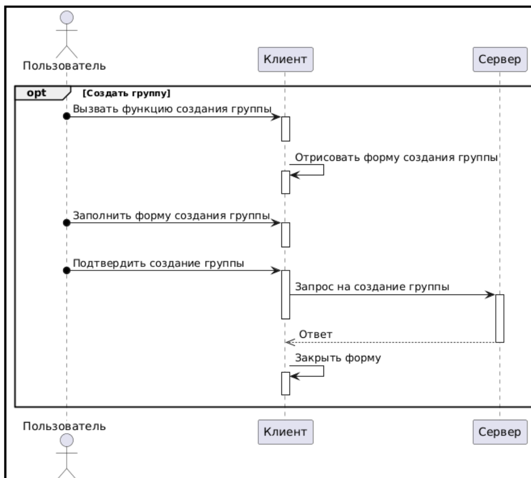
Рисунок 23 - диаграмма последовательности прецедента “Создать группу”
