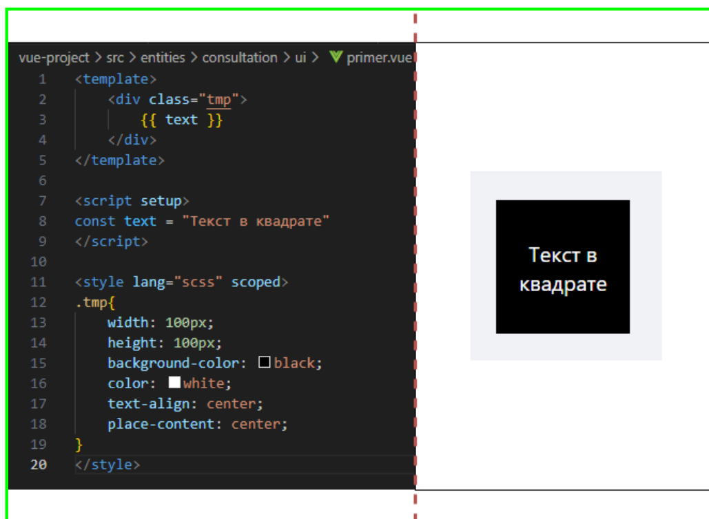
Рисунок 39 – Пример компонента vue
