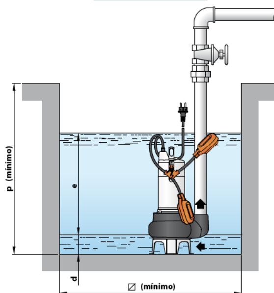
Instalación típica
