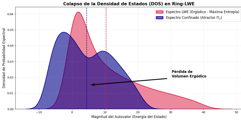
Figure 3. Auditoría termodinámica de la Densidad de Estados (DOS) en el cifrado Ring-LWE. La transición del régimen ergódico asintótico (curva roja) hacia el confinamiento impuesto por el atractor \Pi_2 (curva azul) revela la emergencia de bimodalidad espectral y un desplazamiento restrictivo de la media. Este déficit entrópico certifica analíticamente la ruptura de la Hipótesis de Termalización de los Autoestados (ETH).
