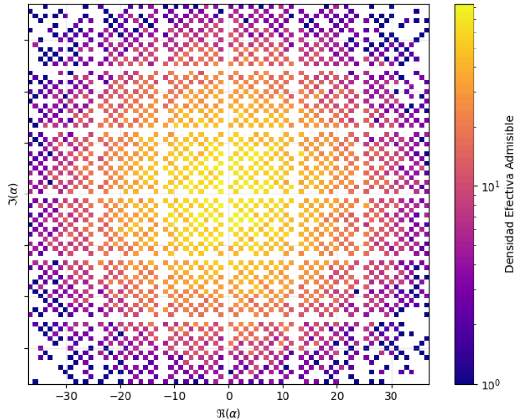
Distribución Condensada Post-Proyección \Pi_2 (Confinamiento de la Celda de Voronoi)
