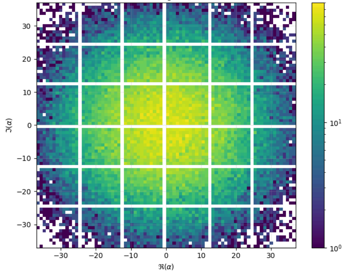
Nube Gaussiana de Ruido (Asunción Ergódica LWE)
