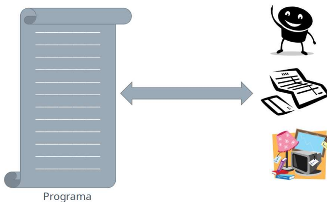
Figura 7.1: Programación estructurada
