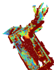
47429736_mono_ft_lidar_all chamfer 12.4 cm, F@5cm 0.29
