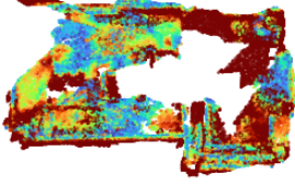
42444474_mono_ft_faro chamfer 10.8 cm, F@5cm 0.31
