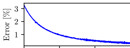
Incoherent
