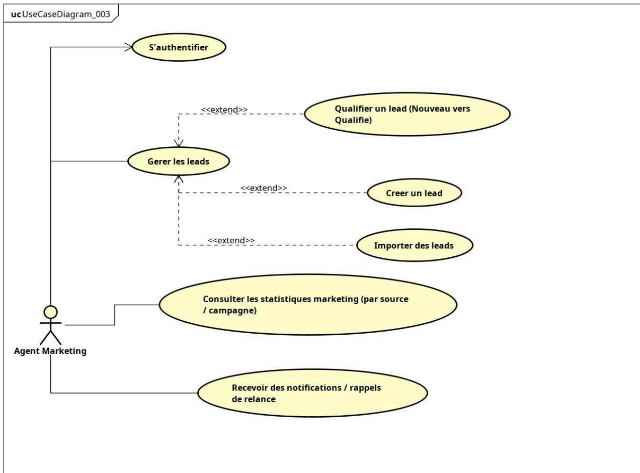
Figure 4 — Diagramme de cas d'utilisation du Tracking Lead System
