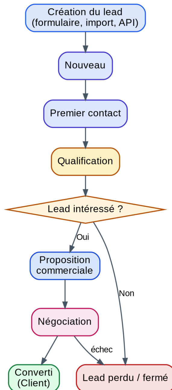
Figure 1 — Cycle de vie d'un lead dans le Tracking Lead System
