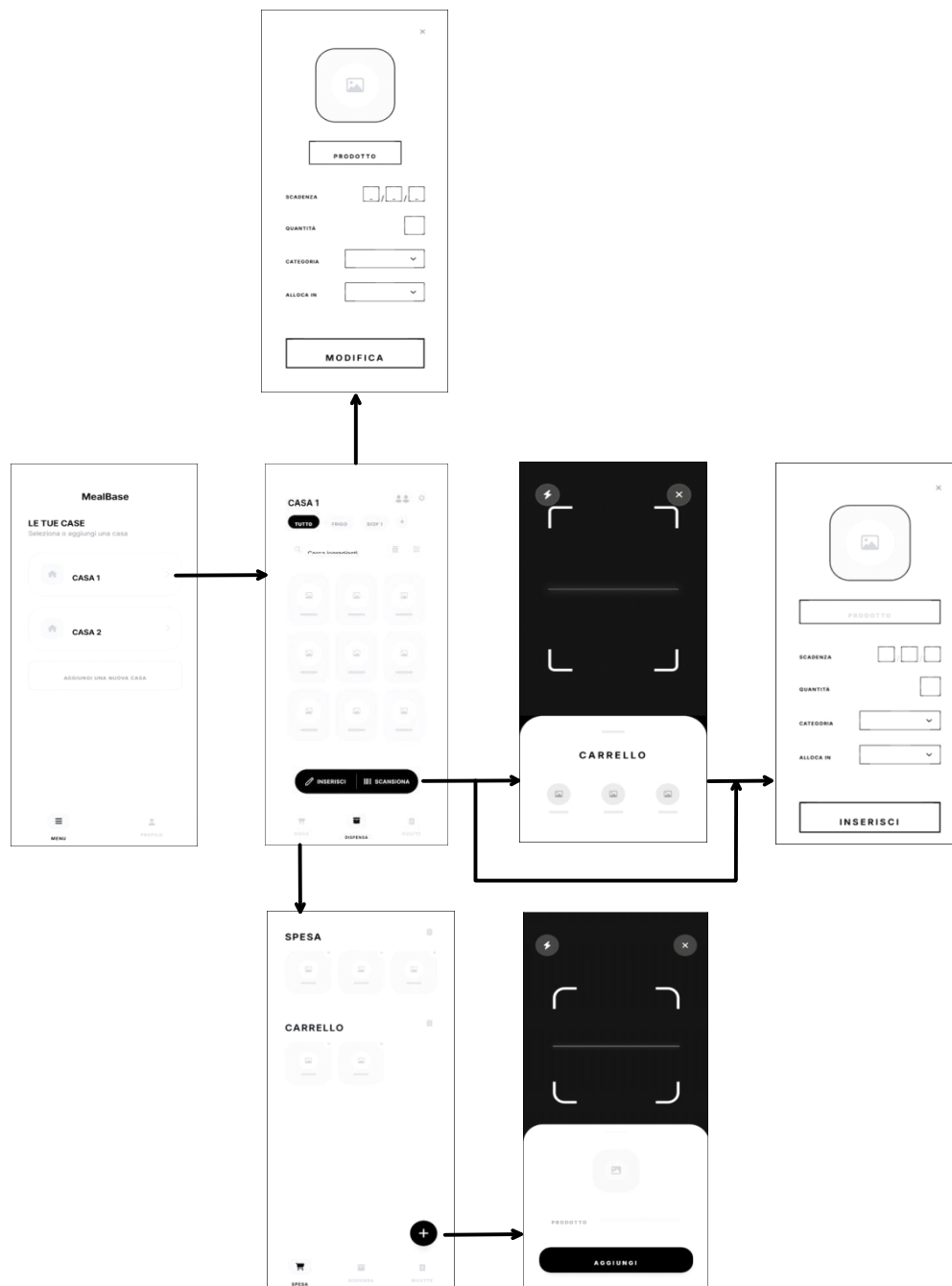
Figure 5: Flusso completo dei wireframe.
