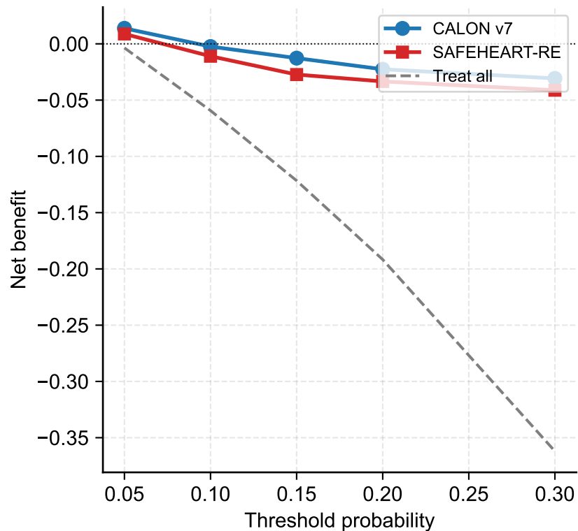
A: Wales→UKB
